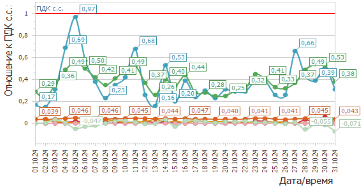
График среднесуточных значений концентраций загрязняющих веществ (в долях ПДК) в атмосферном воздухе в период с 01.10.2024г. по 31.10.2024г. (ПКЗ-3 - автоматическая станция ул.Московская)
