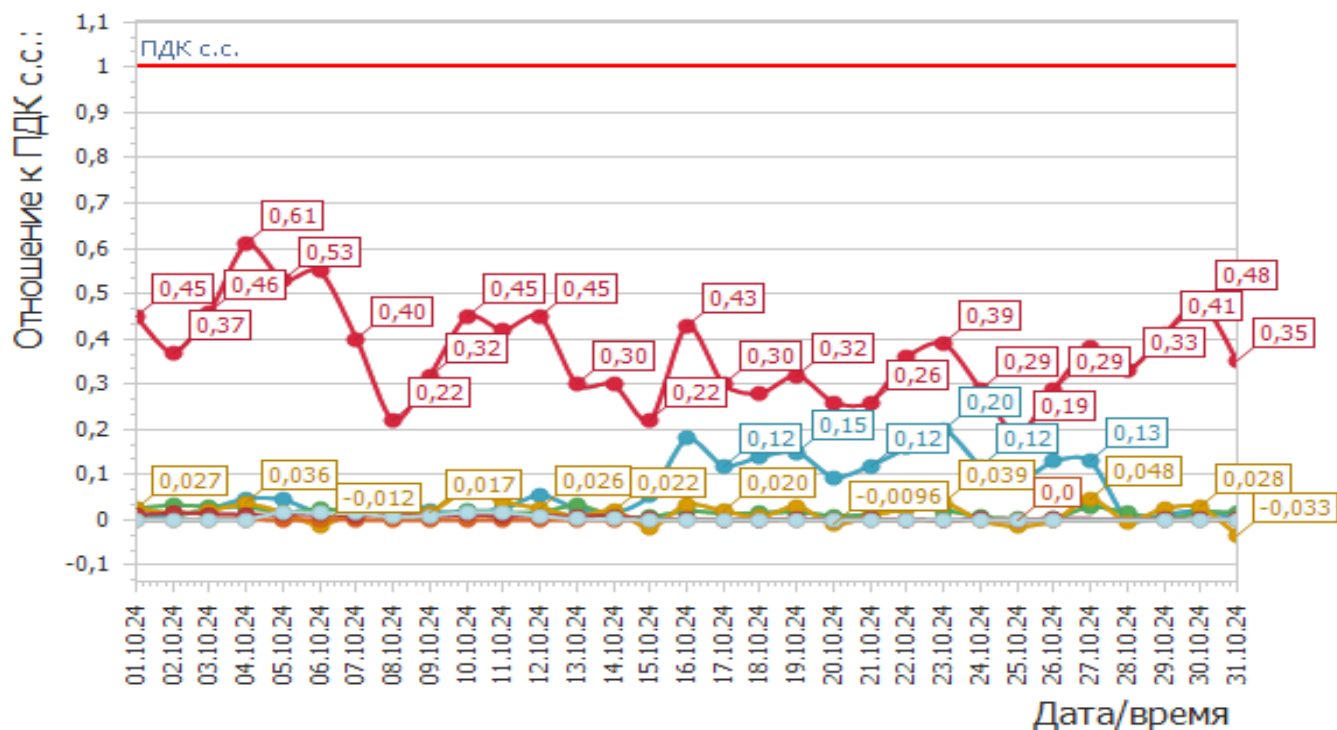
График среднесуточных значений концентраций загрязняющих веществ (в долях ПДК) в атмосферном воздухе в период с 01.10.2024г. по 31.10.2024г. (ПКЗ-1 - автоматическая станция ул.Постовая, 34)
