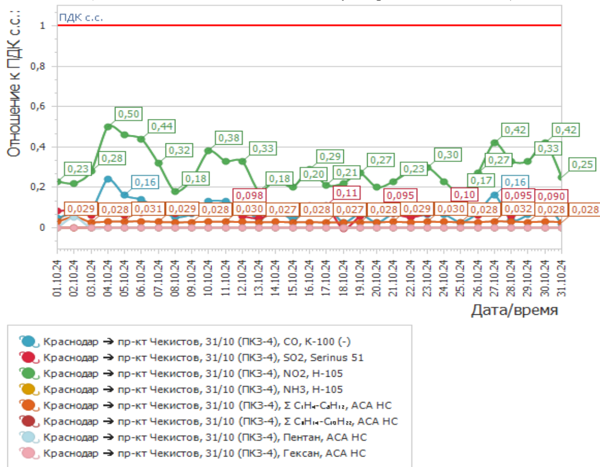
График среднесуточных значений концентраций загрязняющих веществ (мг/м 3 ) в атмосферном воздухе в период с 01.10.2024г. по 31.10.2024г. (ПКЗ 4 - автоматическая станция ул. Проспект Чекистов)
