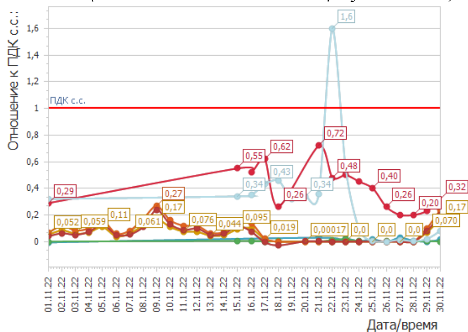
График среднесуточных значений концентраций загрязняющих веществ (в долях ПДК) в атмосферном воздухе в период с 01.11.2022г. по 30.11.2022г. (ПКЗ-1 - автоматическая станция ул. Постовая, 34)
