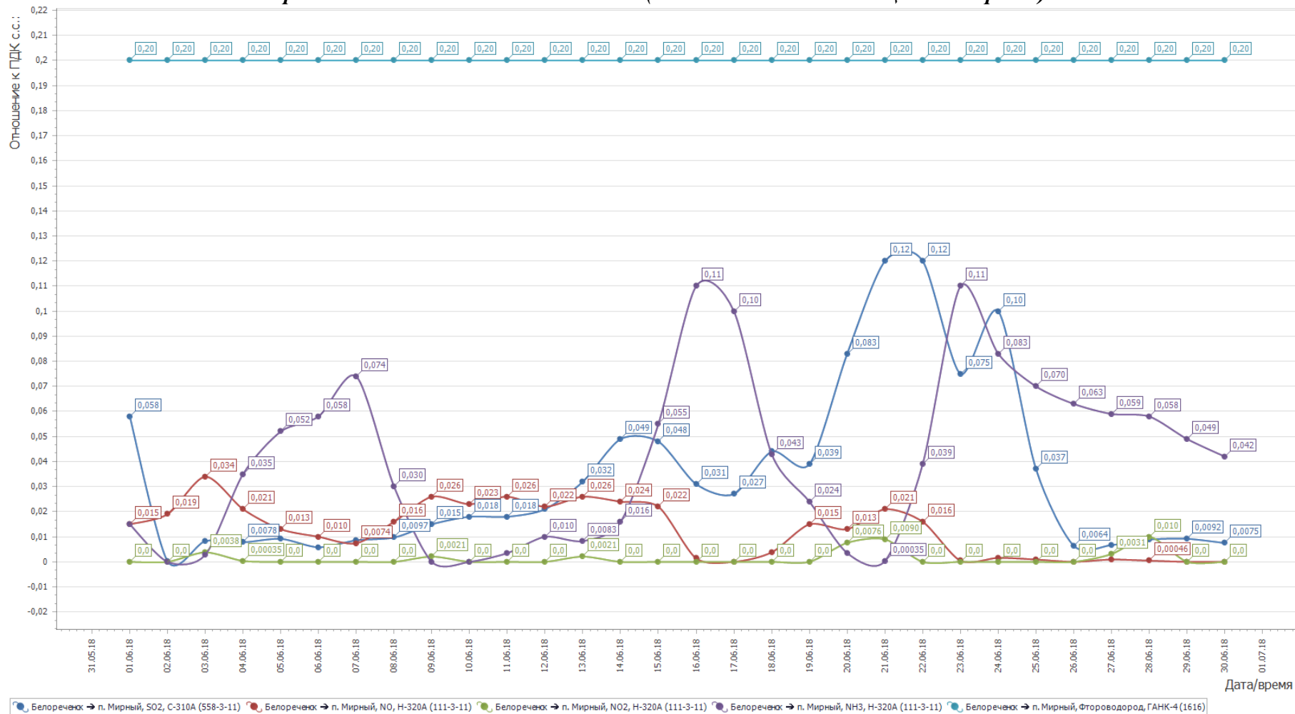
Рисунок 2- График среднесуточных значений концентраций загрязняющих веществ (в долях ПДК) в атмосферном воздухе в период с 01.06.2018г. по 30.06.2018 г. (автоматическая станция п. Мирный)
