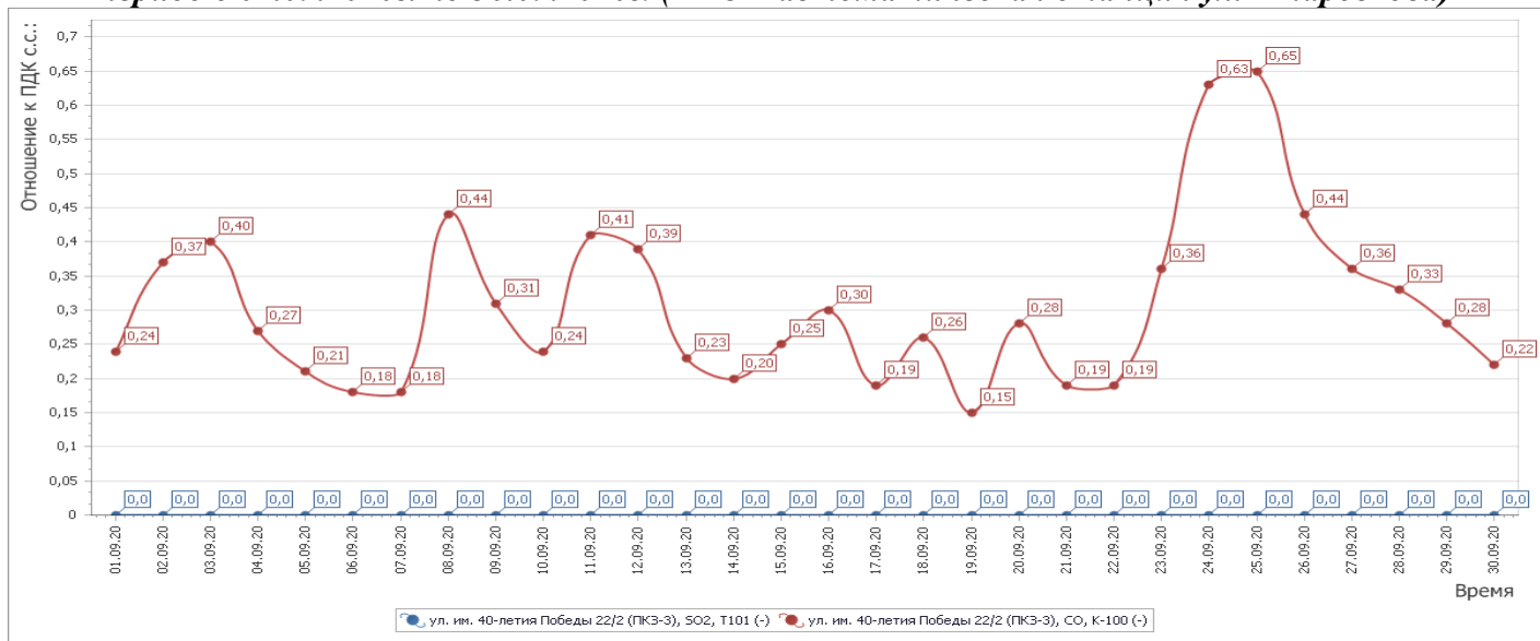
Рисунок 4 - График среднесуточных значений концентраций загрязняющих веществ (в долях ПДК) в атмосферном воздухе в период с 01.09.2020г. по 30.09.2020г. (ПКЗ-2 автоматическая станция ул. Атарбекова)
