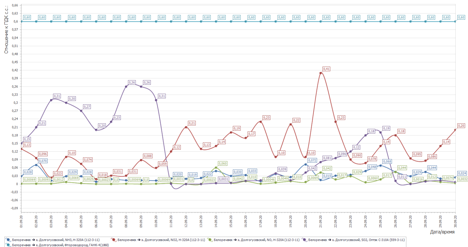
Рисунок 1- График среднесуточных значений концентраций загрязняющих веществ (в долях ПДК) в атмосферном воздухе в период с 01.09.2020г. по 30.09.2020г. (автоматическая станция х. Долгогусевский)
