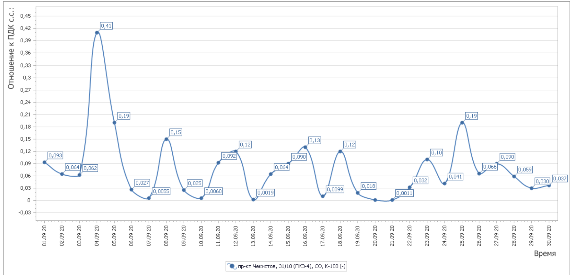
Рисунок 6 - График среднесуточных значений концентраций загрязняющих веществ (в долях ПДК) в атмосферном воздухе в период с 01.09.2020г. по 30.09.2020г. (ПКЗ 4 - автоматическая станция ул. Проспект Чекистов)
