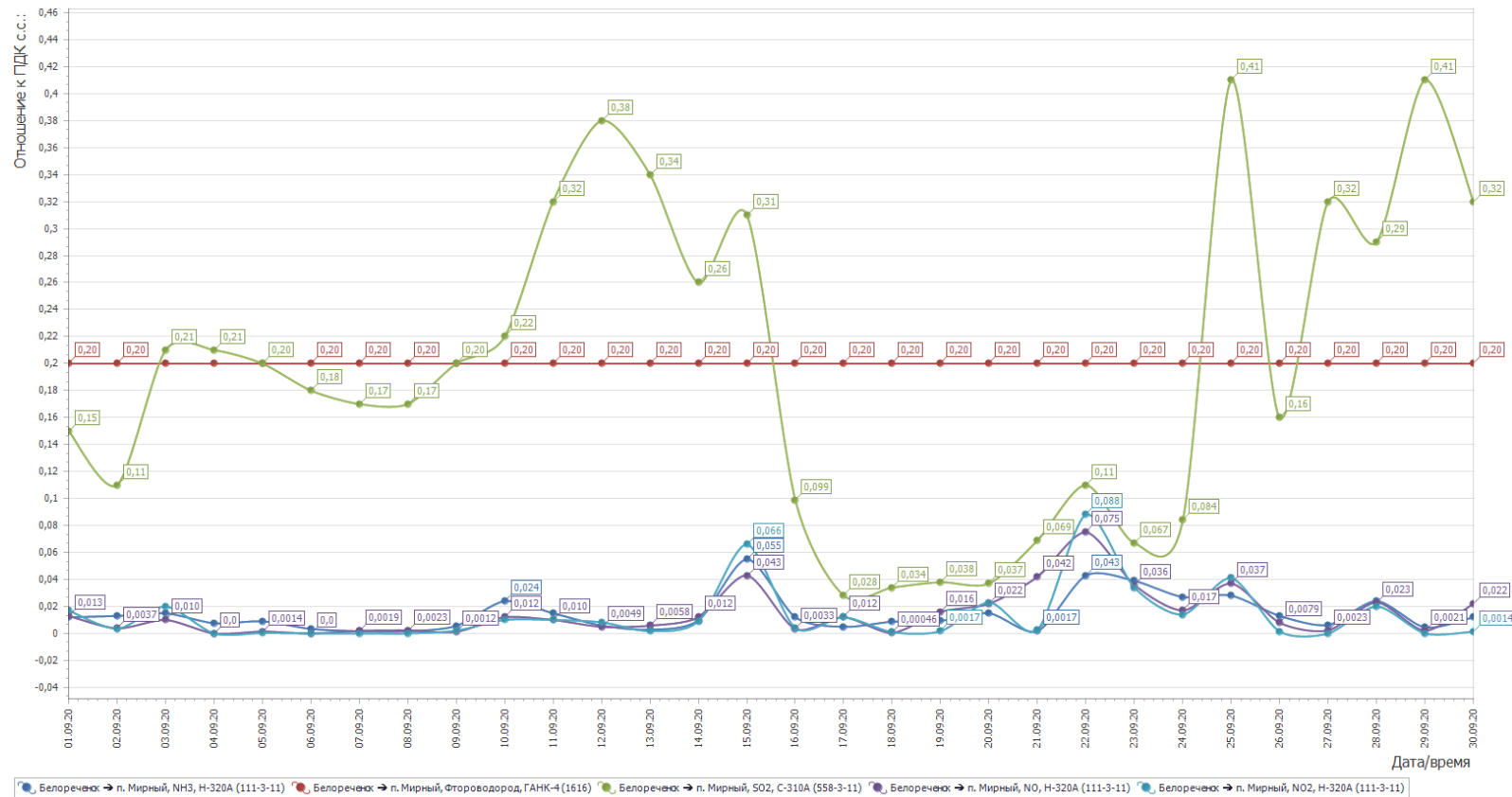
Рисунок 2- График среднесуточных значений концентраций загрязняющих веществ (в долях ПДК) в атмосферном воздухе в период с 01.09.2020г. по 30.09.2020г. (автоматическая станция п. Мирный)
