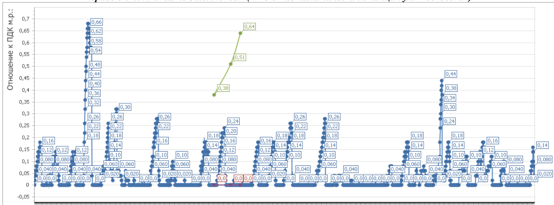
Рисунок 5 - График среднесуточных значений концентраций загрязняющих веществ (в долях ПДК) в атмосферном воздухе в период с 01.09.2020г. по 30.09.2020г. (ПКЗ-3 - автоматическая станция ул. Московская)
