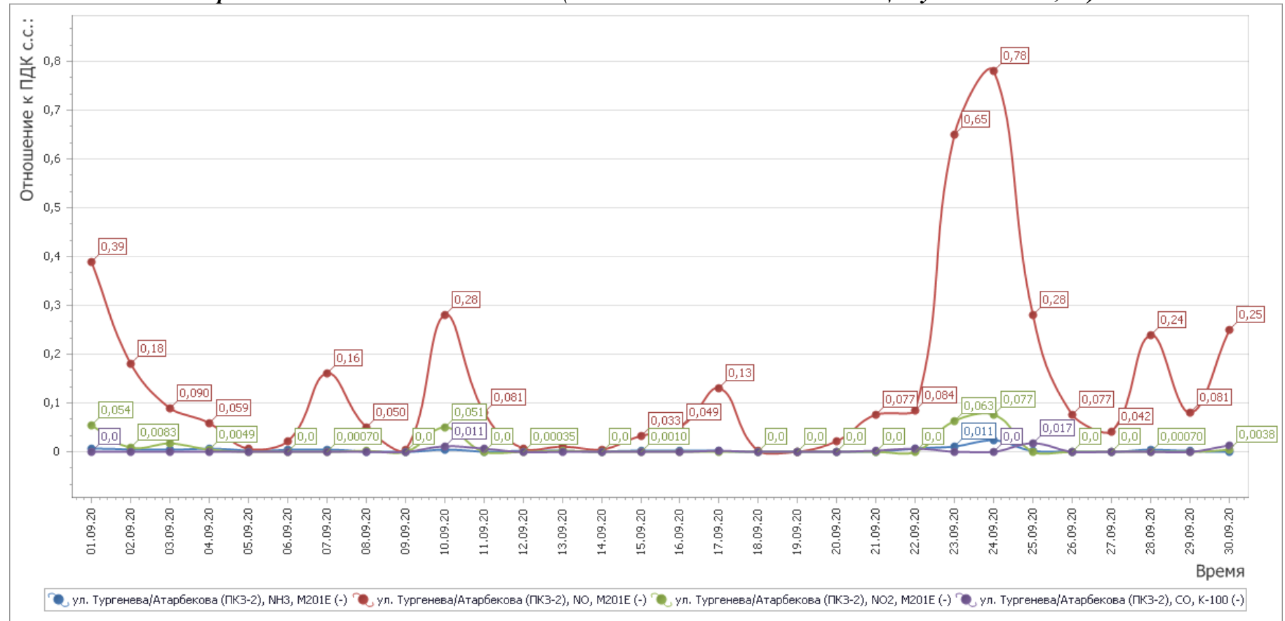
Рисунок 3- График среднесуточных значений концентраций загрязняющих веществ (в долях ПДК) в атмосферном воздухе в период с 01.09.2020г. по 30.09.2020г. (ПКЗ-1 - автоматическая станция ул. Постовая, 34)
