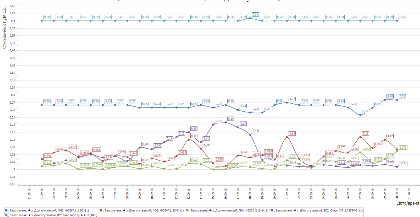
Рисунок 1- График среднесуточных значений концентраций загрязняющих веществ (в долях ПДК ) в атмосферном воздухе в период с 01.09.2018г. по 30.09.2018 г. (автоматическая станция х. Долгогусевский)
