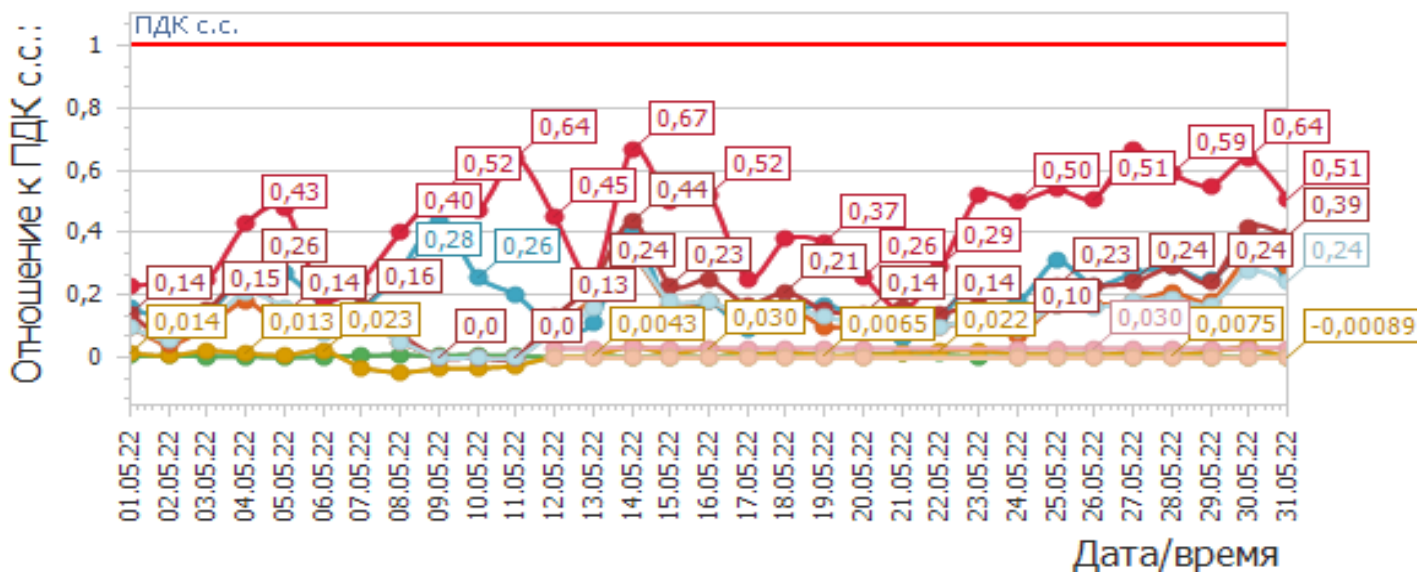
График среднесуточных значений концентраций загрязняющих веществ (в долях ПДК) в атмосферном воздухе в период с 01.05.2022г. по 31.05.2022г. (ПКЗ-3 - автоматическая станция ул.Московская)
