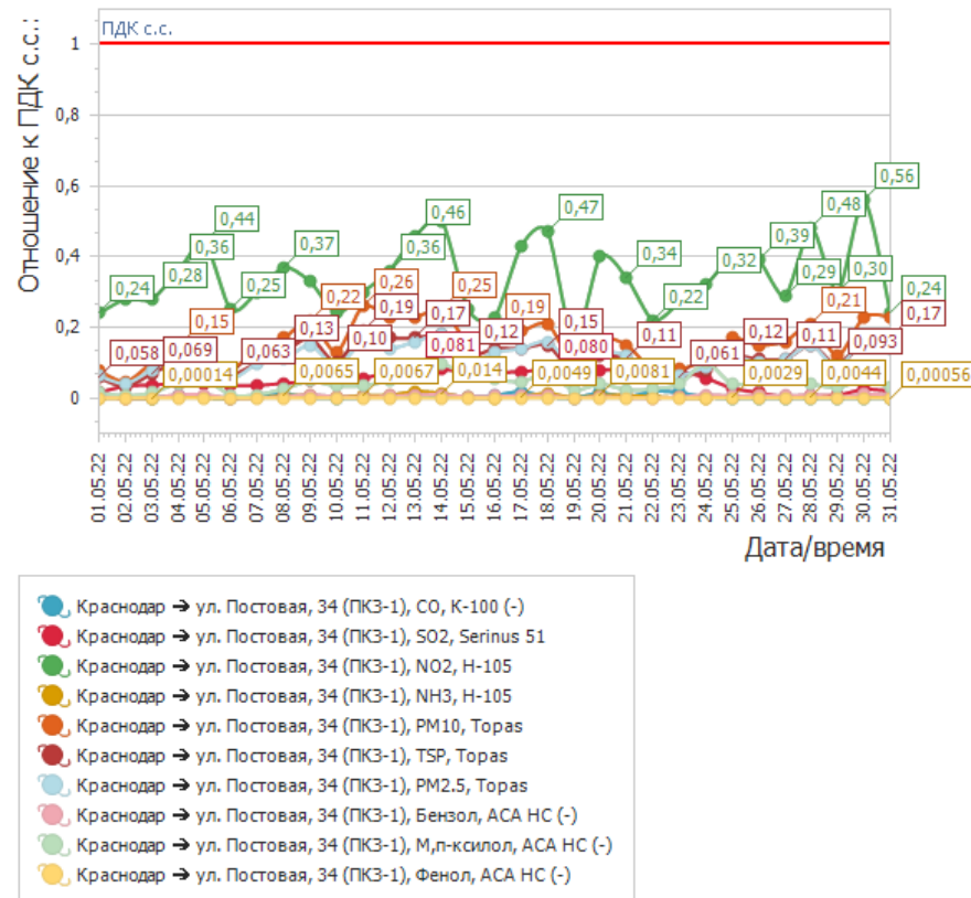
График среднесуточных значений концентраций загрязняющих веществ (в долях ПДК) в атмосферном воздухе в период с 01.05.2022г. по 31.05.2022г. (ПКЗ-1 - автоматическая станция ул.Пастуховая, 34)
