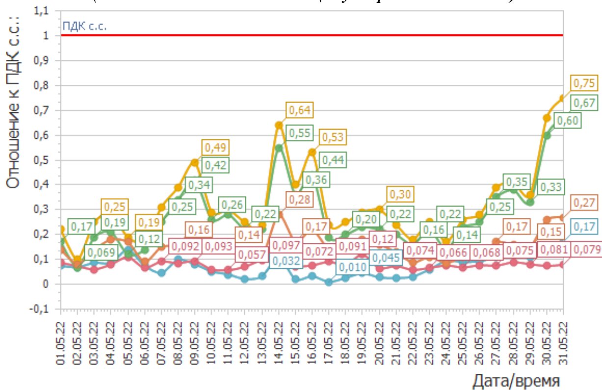
График среднесуточных значений концентраций загрязняющих веществ (мг/м 3 ) в атмосферном воздухе в период 01.05.2022г. по 31.05.2022г. (ПКЗ 4 - автоматическая станция ул. Проспект Чекистов)
