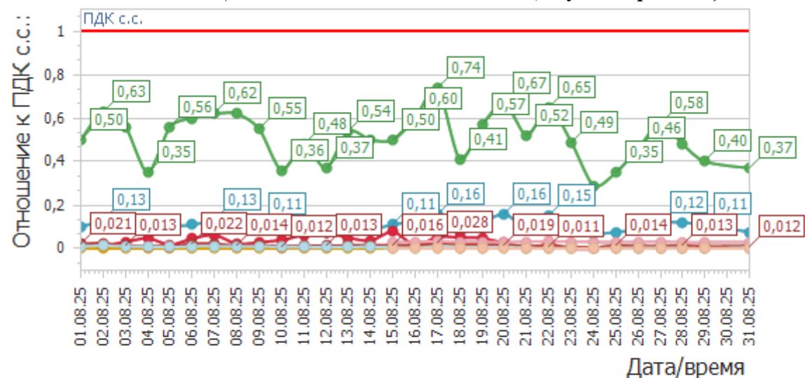
График среднесуточных значений концентраций загрязняющих веществ (мг/м³) в атмосферном воздухе в период с 01.08.2025г. по 31.08.2025г. (ПКЗ-2 автоматическая станция ул.Атарбекова)
