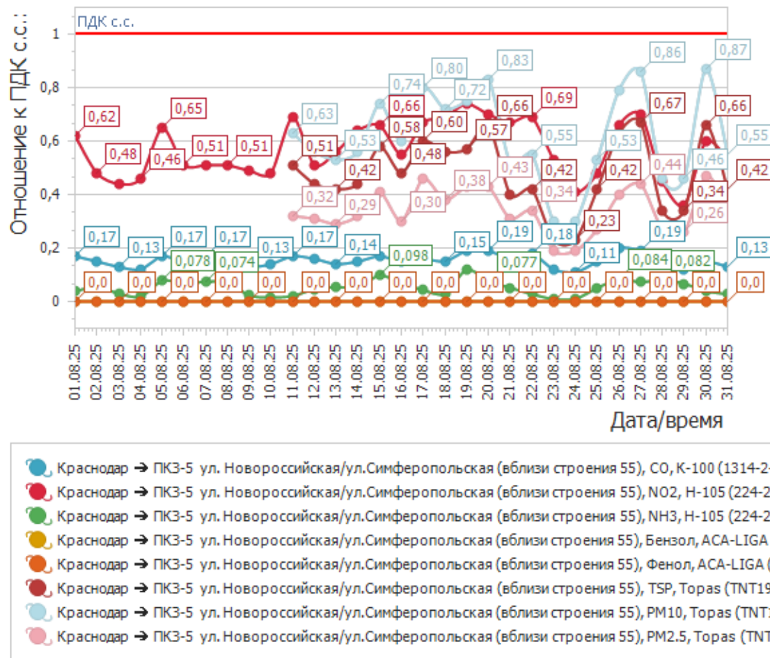
График среднесуточных значений концентраций загрязняющих веществ (мг/м³) в атмосферном воздухе в период с 01.08.2025 г. по 31.08.2025 г. (ПКЗ 5 - ул.Новороссийская/ул.Симферопольская вблизи строения 55)
