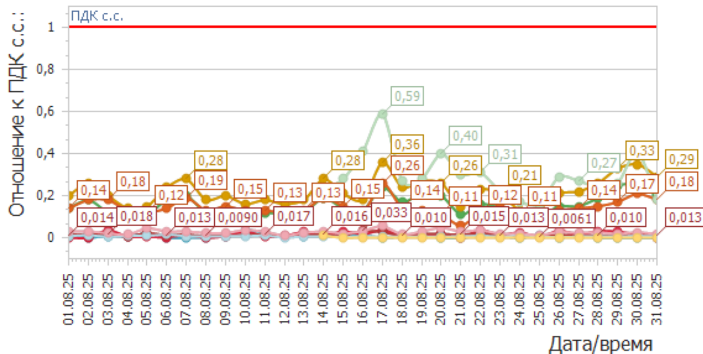
График среднесуточных значений концентраций загрязняющих веществ (в долях ПДК) в атмосферном воздухе в период с 01.08.2025г. по 31.08.2025г. (ПКЗ-1 - автоматическая станция ул.Постовая, 34)
