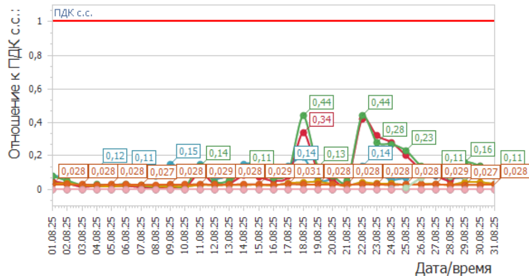
График среднесуточных значений концентраций загрязняющих веществ (мг/м 3 ) в атмосферном воздухе в период с 01.08.2025г. по 31.08.2025г. (ПКЗ 4 - автоматическая станция ул. Проспект Чекистов)
