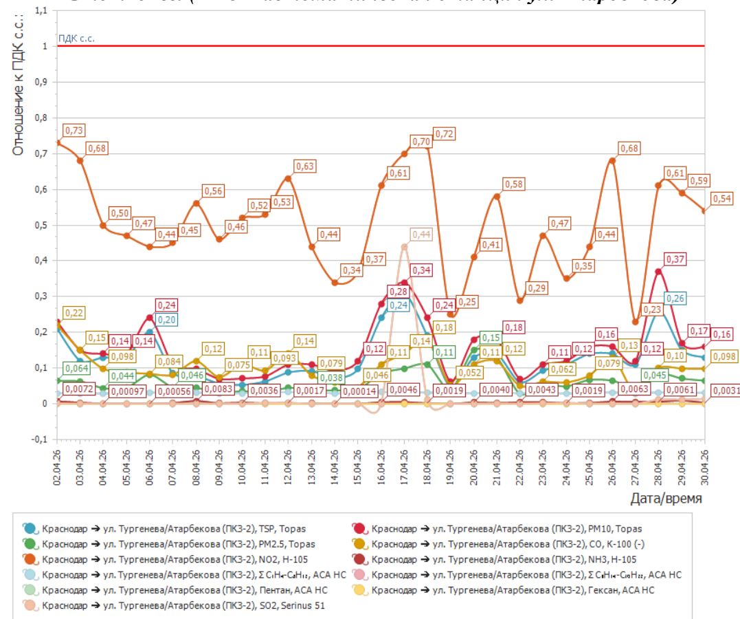
График среднесуточных значений концентраций загрязняющих веществ ( \text{мг}/\text{м}^3 ) в атмосферном воздухе в период с 01.04.2026г. по 31.04.2026г. (ПКЗ-2 автоматическая станция ул.Атарбекова)
