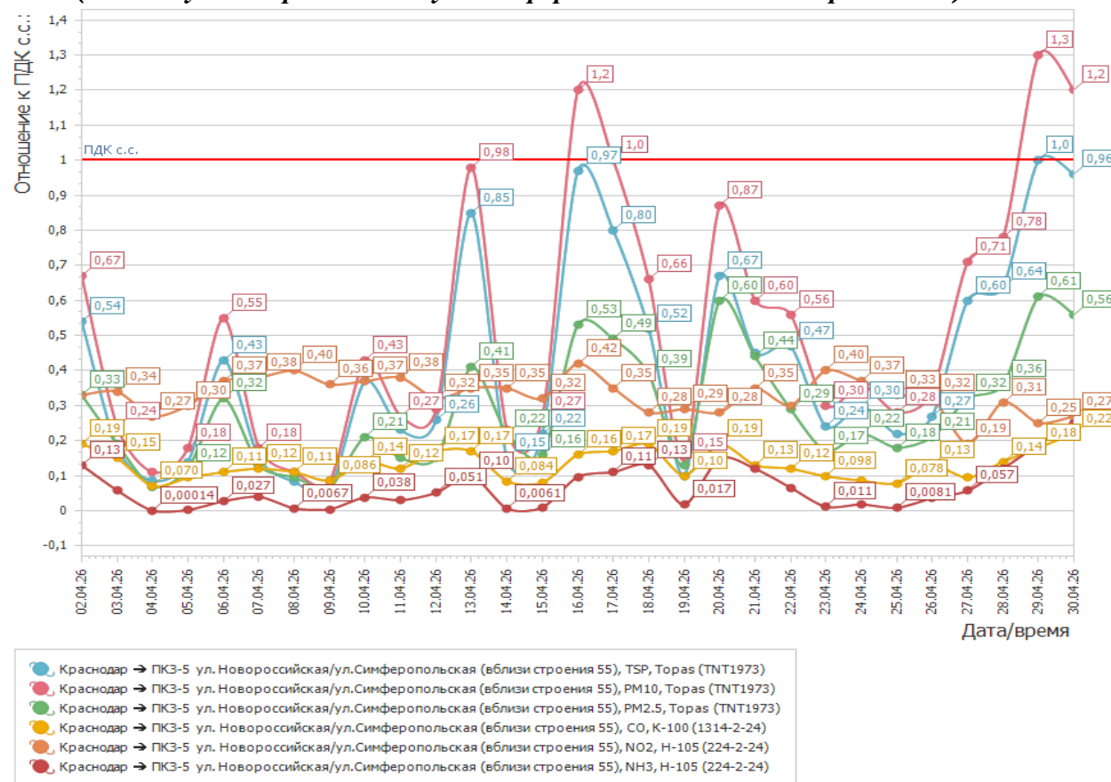
График среднесуточных значений концентраций загрязняющих веществ ( \text{мг}/\text{м}^3 ) в атмосферном воздухе в период 01.04.2026г. по 30.04.2026г. (ПКЗ 5 - ул.Новороссийская/ул.Симферопольская вблизи строения 55)
