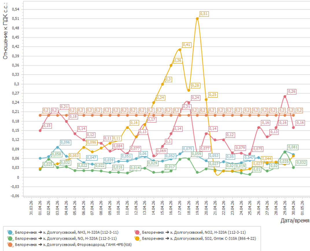
График среднесуточных значений концентраций загрязняющих веществ (в долях ПДК) в атмосферном воздухе в период с 01.04.2026г. по 30.04.2026г. (автоматическая станция х. Долгогусевский)
