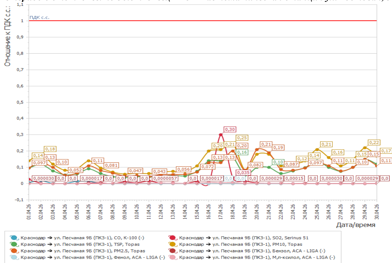
График среднесуточных значений концентраций загрязняющих веществ (в долях ПДК) в атмосферном воздухе в период с 01.04.2026г. по 30.04.2026г. (ПКЗ-1 - автоматическая станция ул.Постовая, 34)
