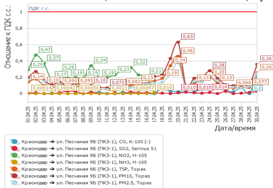
График среднесуточных значений концентраций загрязняющих веществ (в долях ПДК) в атмосферном воздухе в период с 01.04.2025г. по 30.04.2025г.(ПКЗ-1 - автоматическая станция ул.Пестовая, 34)
