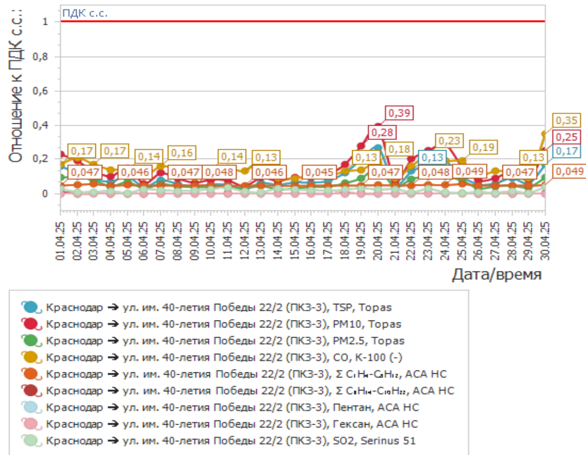
График среднесуточных значений концентраций загрязняющих веществ (в долях ПДК) в атмосферном воздухе в период с 01.04.2025г. по 30.04.2025г. (ПКЗ-3 - автоматическая станция ул.Московская)
