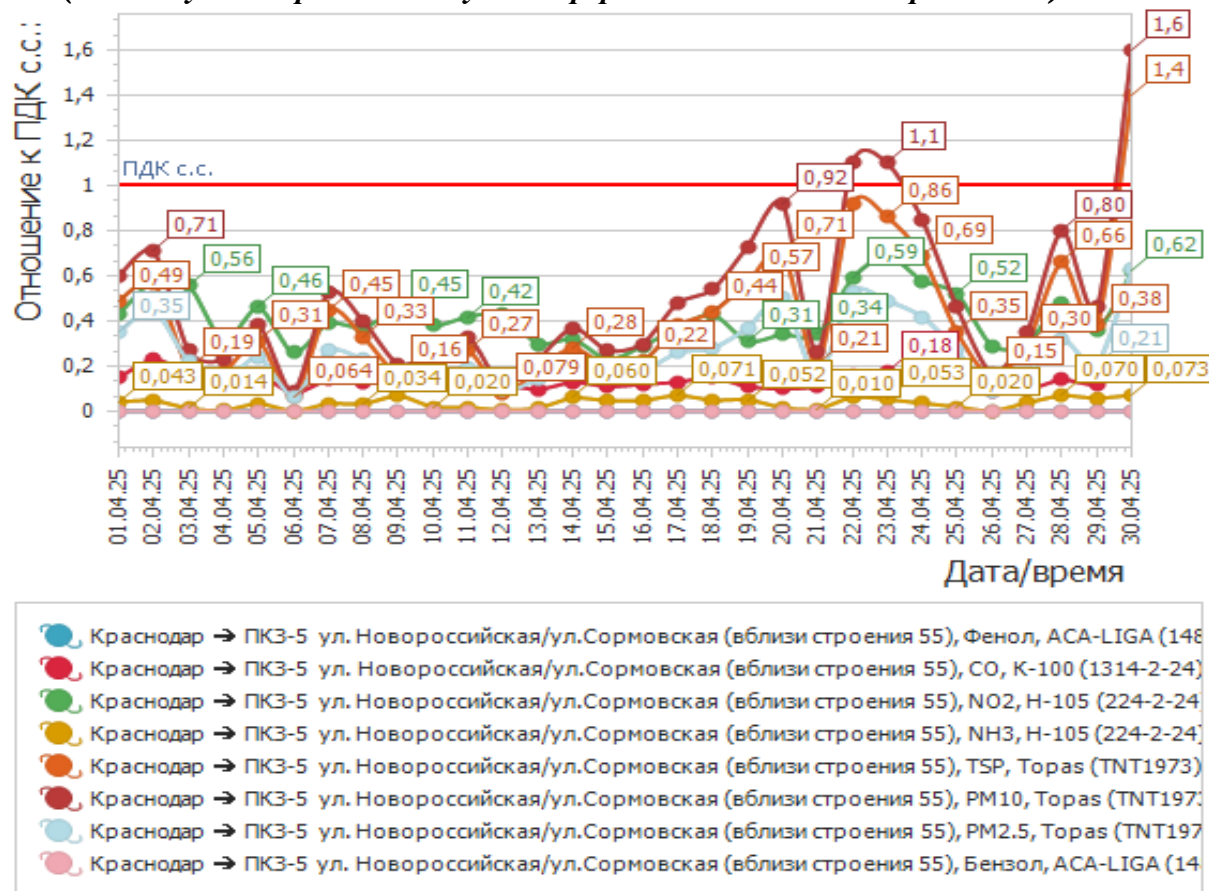
График среднесуточных значений концентраций загрязняющих веществ (мг/м³) в атмосферном воздухе в период 01.04.2025г. по 30.04.2025г. (ПКЗ 5 - ул.Новороссийская/ул.Симферопольская вблизи строения 55)
