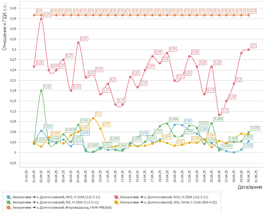
График среднесуточных значений концентраций загрязняющих веществ (в долях ПДК) в атмосферном воздухе в период с 01.04.2025г. по 30.04.2025г. (автоматическая станция х. Долгогусевский)
