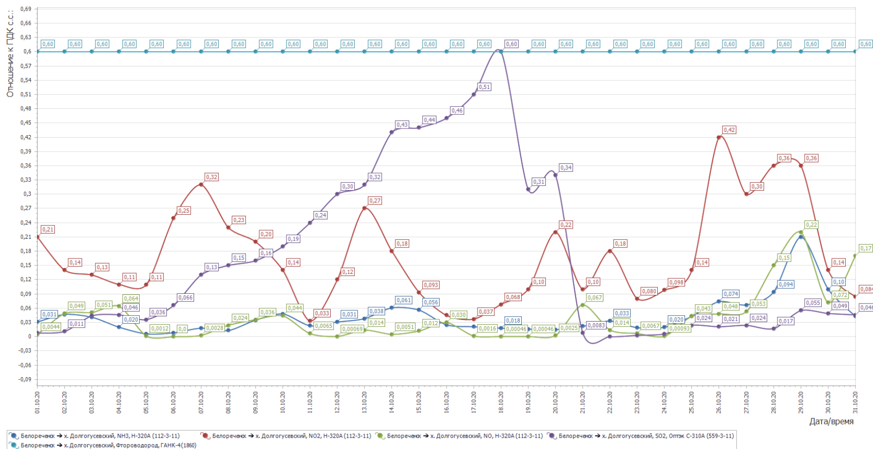
Рисунок 1- График среднесуточных значений концентраций загрязняющих веществ (в долях ПДК) в атмосферном воздухе в период с 01.10.2020г. по 31.10.2020г. (автоматическая станция х. Долгогусевский)
