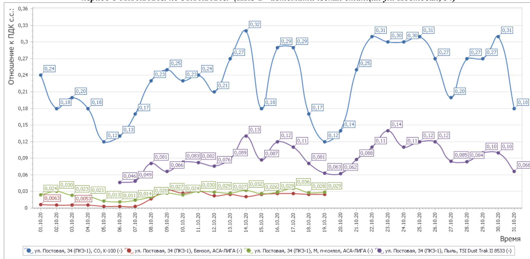
Рисунок 3- График среднесуточных значений концентраций загрязняющих веществ (в долях ПДК) в атмосферном воздухе в период с 01.10.2020г. по 31.10.2020г. (ПКЗ-1 - автоматическая станция ул. Постовая, 34)
