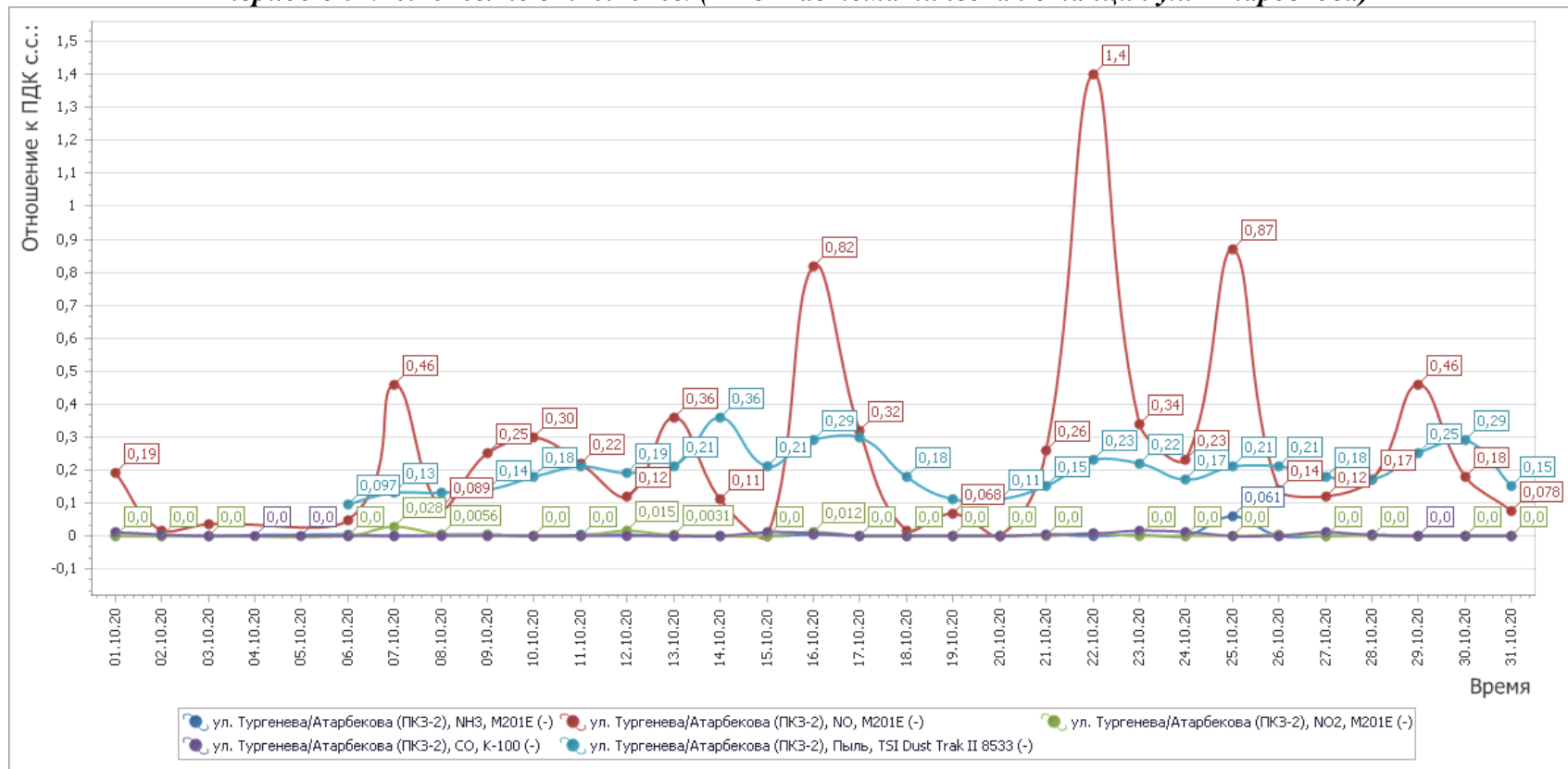
Рисунок 4 - График среднесуточных значений концентраций загрязняющих веществ (в долях ПДК) в атмосферном воздухе в период с 01.10.2020г. по 31.10.2020г. (ПКЗ-2 автоматическая станция ул. Атарбекова)
