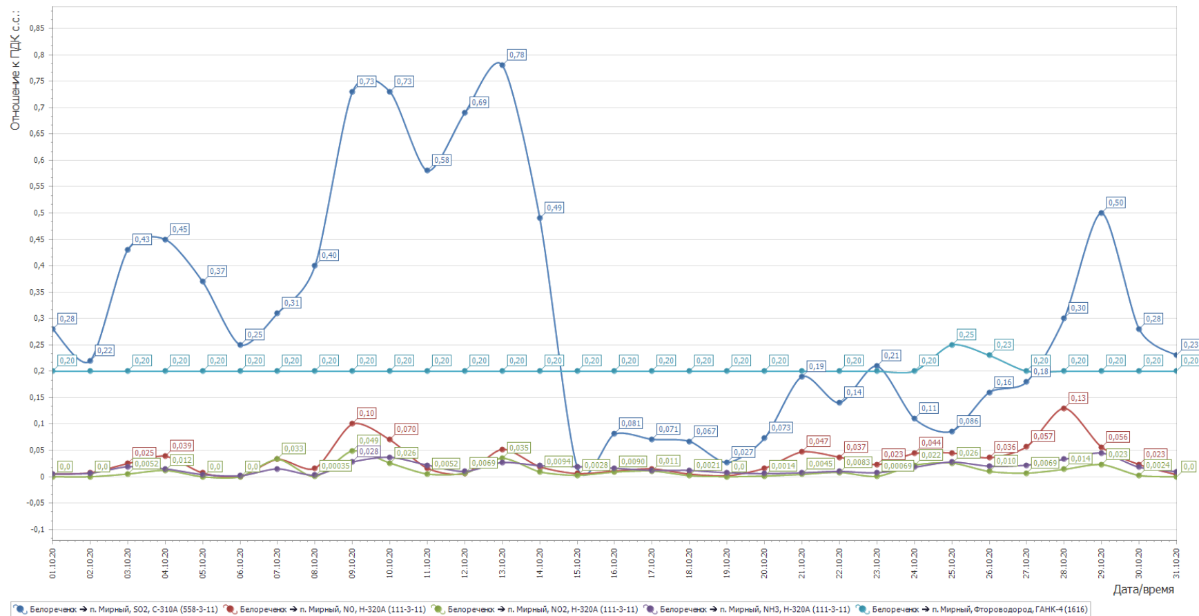
Рисунок 2- График среднесуточных значений концентраций загрязняющих веществ (в долях ПДК) в атмосферном воздухе в период с 01.10.2020г. по 31.10.2020г. (автоматическая станция п. Мирный)
