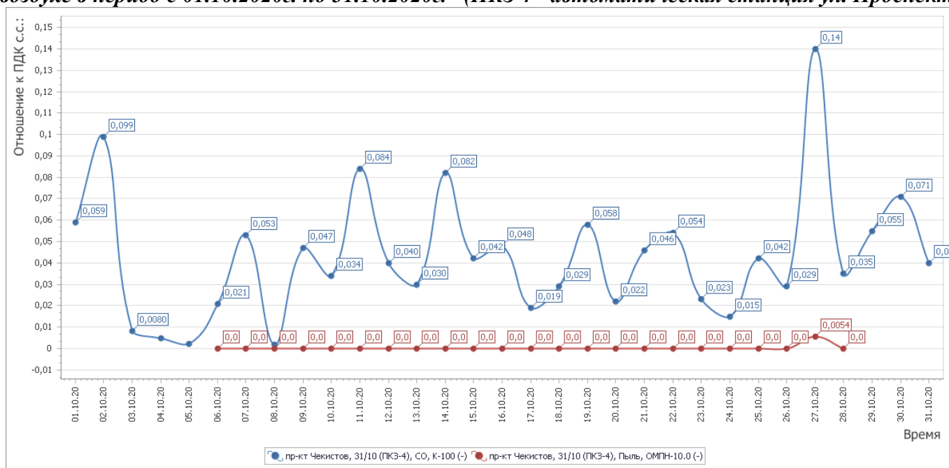
Рисунок 6 - График среднесуточных значений концентраций загрязняющих веществ (в долях ПДК) в атмосферном воздухе в период с 01.10.2020г. по 31.10.2020г. (ПКЗ 4 - автоматическая станция ул. Проспект Чекистов)
