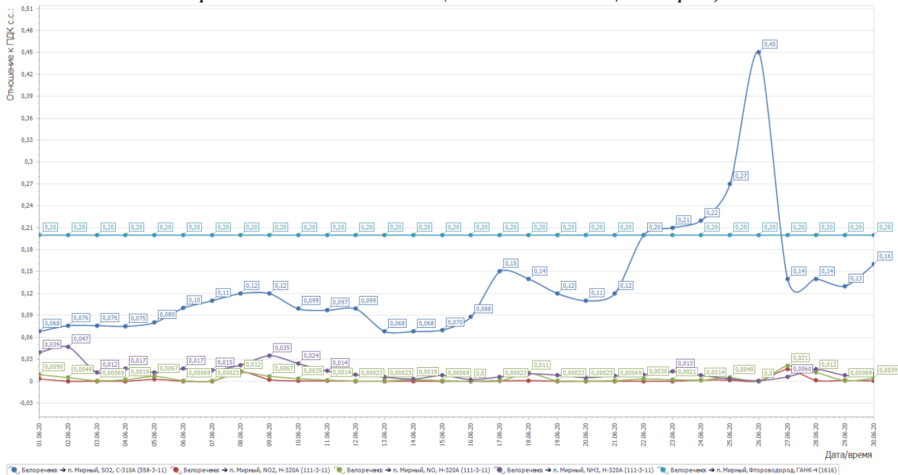
Рисунок 2- График среднесуточных значений концентраций загрязняющих веществ (в долях ПДК) в атмосферном воздухе в период с 01.06.2020г. по 30.06.2020г. (автоматическая станция п. Мирный)
