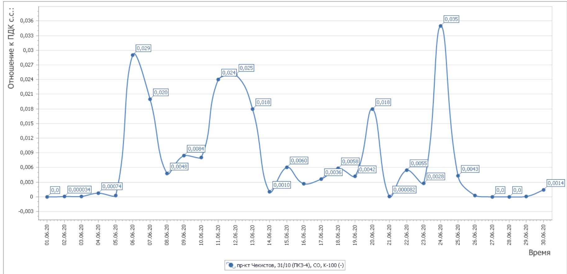
Рисунок 6 - График среднесуточных значений концентраций загрязняющих веществ (в долях ПДК) в атмосферном воздухе в период с 01.06.2020г. по 30.06.2020г. (ПКЗ 4 - автоматическая станция ул. Проспект Чекистов)
