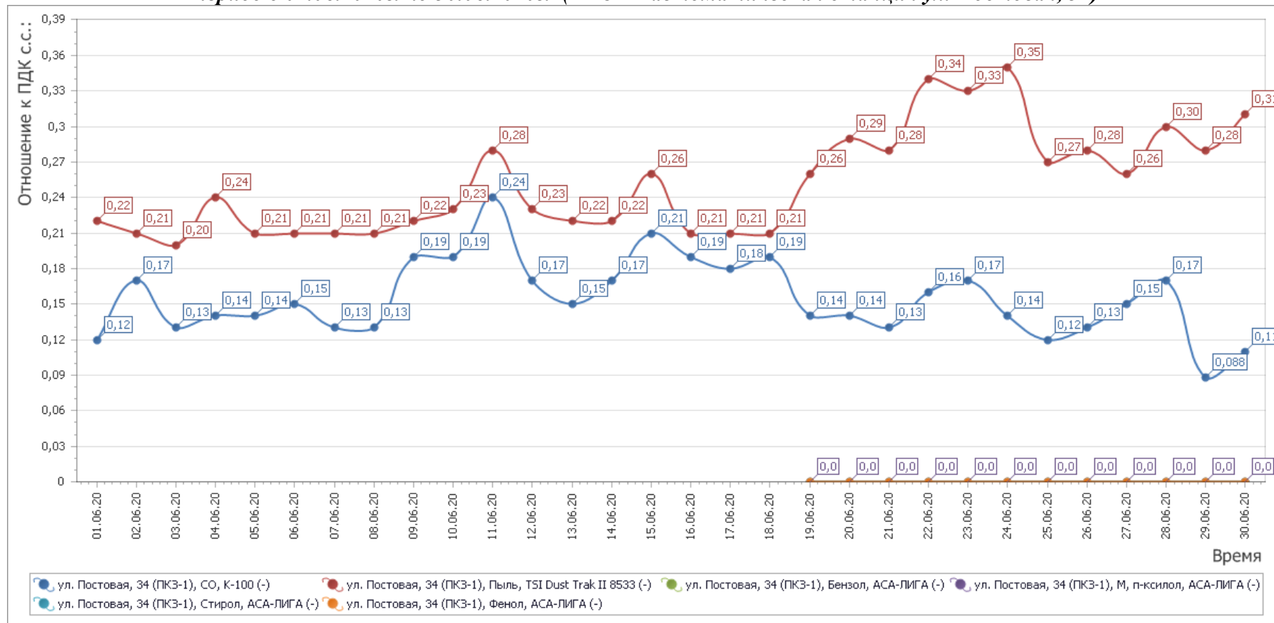
Рисунок 3- График среднесуточных значений концентраций загрязняющих веществ (в долях ПДК) в атмосферном воздухе в период с 01.06.2020г. по 30.06.2020г. (ПКЗ-1 - автоматическая станция ул. Постовая, 34)
