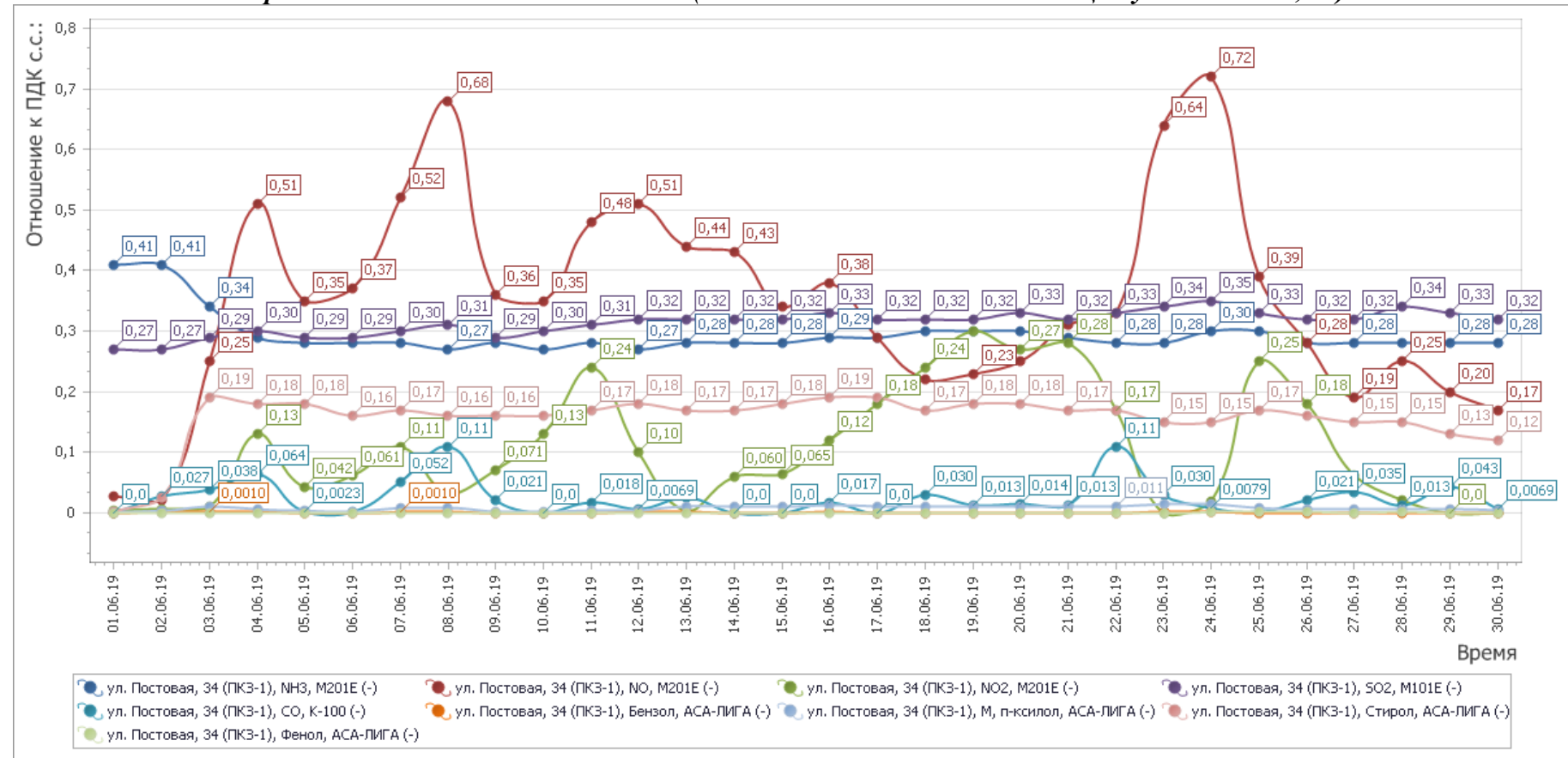
Рисунок 3- График среднесуточных значений концентраций загрязняющих веществ (в долях ПДК) в атмосферном воздухе в период с 01.06.2019г. по 30.06.2019 г. (ПКЗ-1 - автоматическая станция ул. Постовая, 34)
