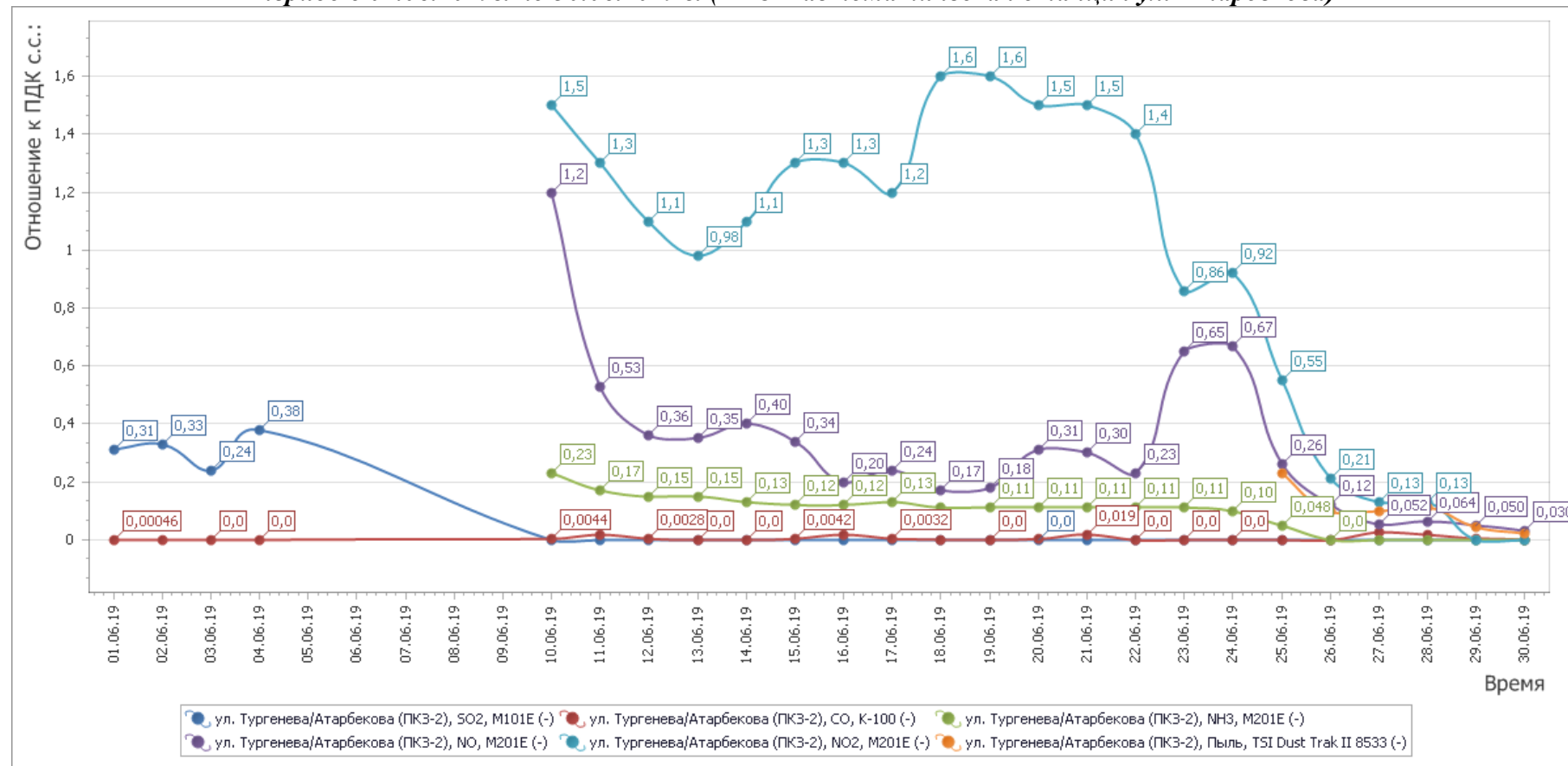
Рисунок 4 - График среднесуточных значений концентраций загрязняющих веществ (в долях ПДК) в атмосферном воздухе в период с 01.06.2019г. по 30.06.2019 г. (ПКЗ-2 автоматическая станция ул. Атарбекова)
