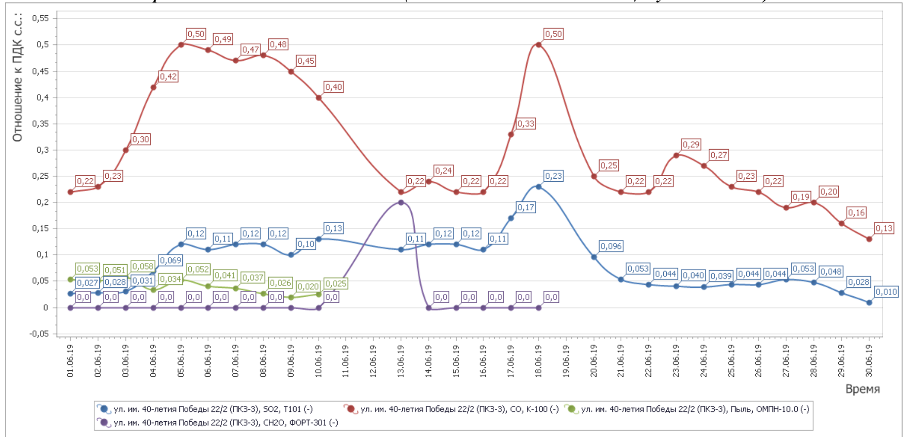
Рисунок 5 - График среднесуточных значений концентраций загрязняющих веществ (в долях ПДК) в атмосферном воздухе в период с 01.06.2019 г. по 30.06.2019 г. (ПКЗ-3 - автоматическая станция ул. Московская)
