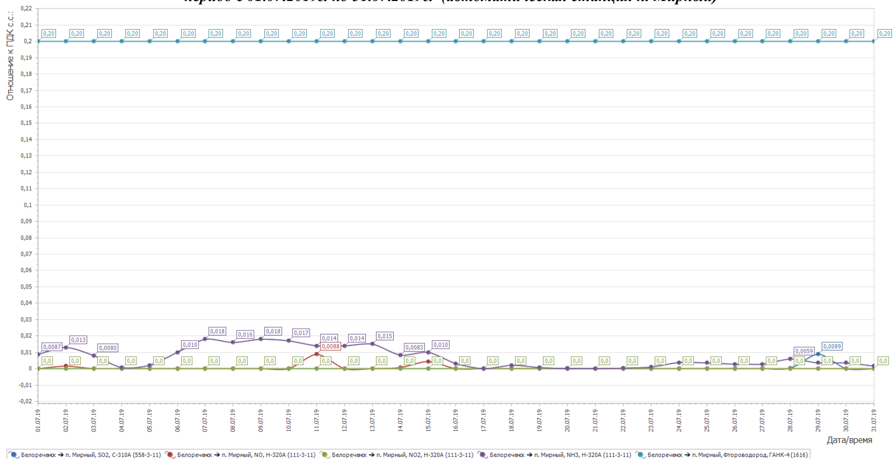
Рисунок 2- График среднесуточных значений концентраций загрязняющих веществ (в долях ПДК) в атмосферном воздухе в период с 01.07.2019г. по 31.07.2019г. (автоматическая станция п. Мирный)
