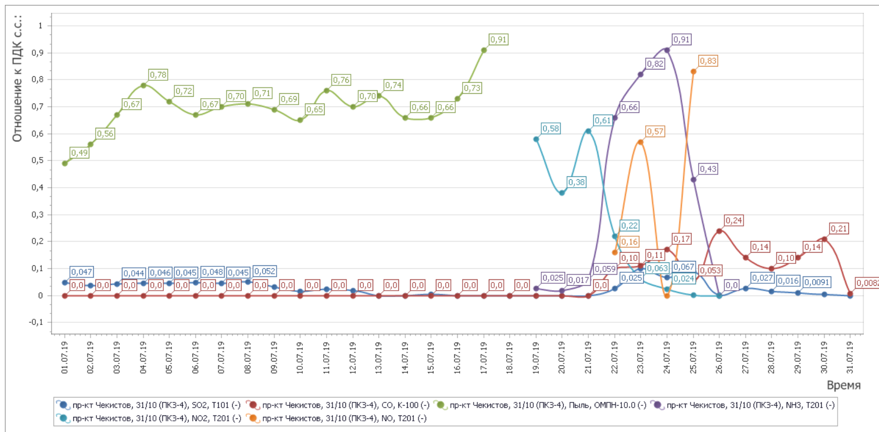
Рисунок 6 - График среднесуточных значений концентраций загрязняющих веществ (в долях ПДК) в атмосферном воздухе в период с 01.07.2019г. по 31.07.2019 г. (ПКЗ 4 - автоматическая станция ул. Проспект Чекистов)
