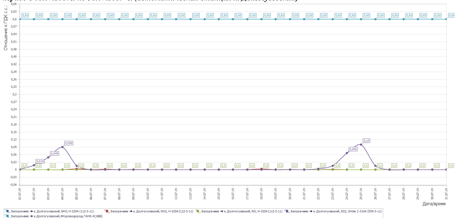
Рисунок 1- График среднесуточных значений концентраций загрязняющих веществ (в долях ПДК) в атмосферном воздухе в период с 01.07.2019г. по 31.07.2019 г. (автоматическая станция х. Долгогусевский)
