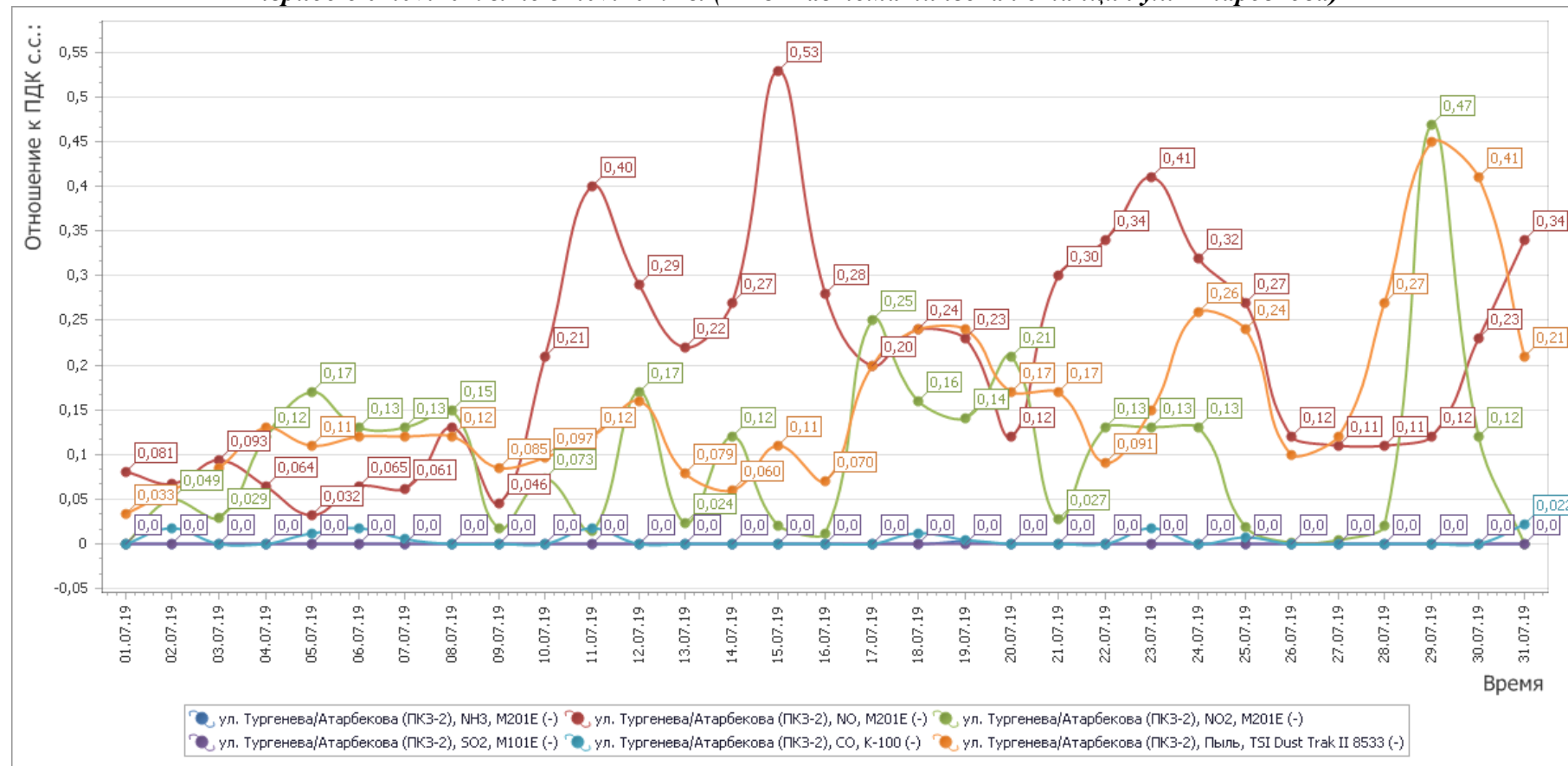
Рисунок 4 - График среднесуточных значений концентраций загрязняющих веществ (в долях ПДК) в атмосферном воздухе в период с 01.07.2019г. по 31.07.2019 г. (ПКЗ-2 автоматическая станция ул. Атарбекова)
