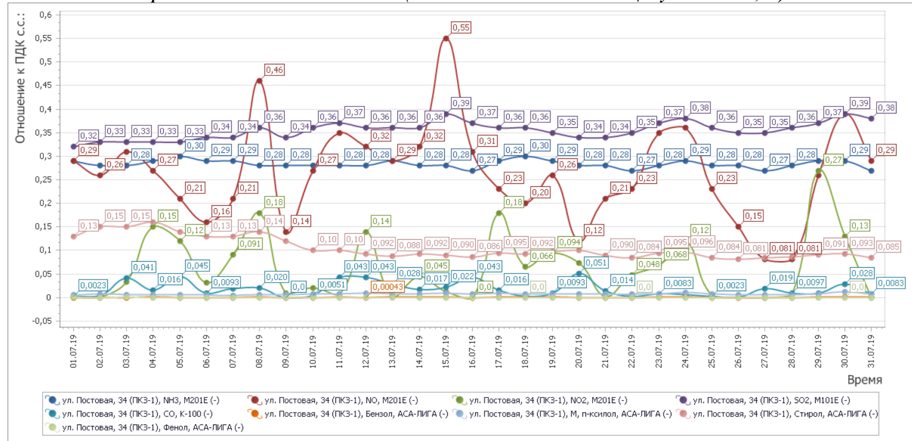
Рисунок 3- График среднесуточных значений концентраций загрязняющих веществ (в долях ПДК) в атмосферном воздухе в период с 01.07.2019г. по 31.07.2019 г. (ПКЗ-1 - автоматическая станция ул. Постовая, 34)
