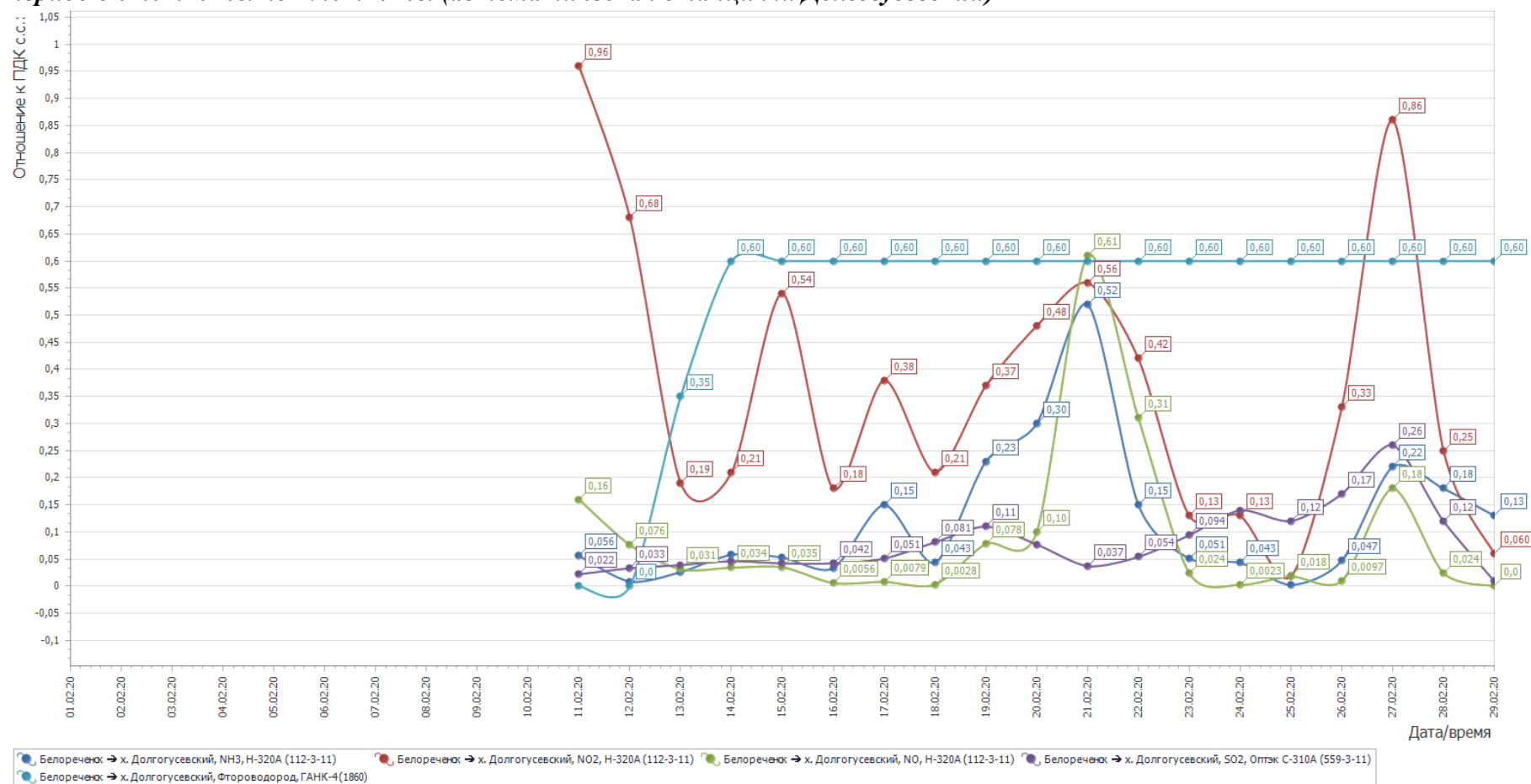
Рисунок 1- График среднесуточных значений концентраций загрязняющих веществ (в долях ПДК) в атмосферном воздухе в период с 01.02.2020г. по 29.02.2020г. (автоматическая станция х. Долгогусевский)
