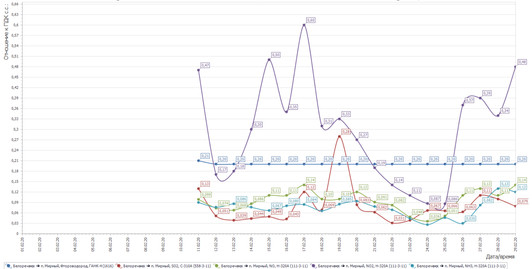
Рисунок 2- График среднесуточных значений концентраций загрязняющих веществ (в долях ПДК) в атмосферном воздухе в период с 01.02.2020г. по 29.02.2020г. (автоматическая станция п. Мирный)
