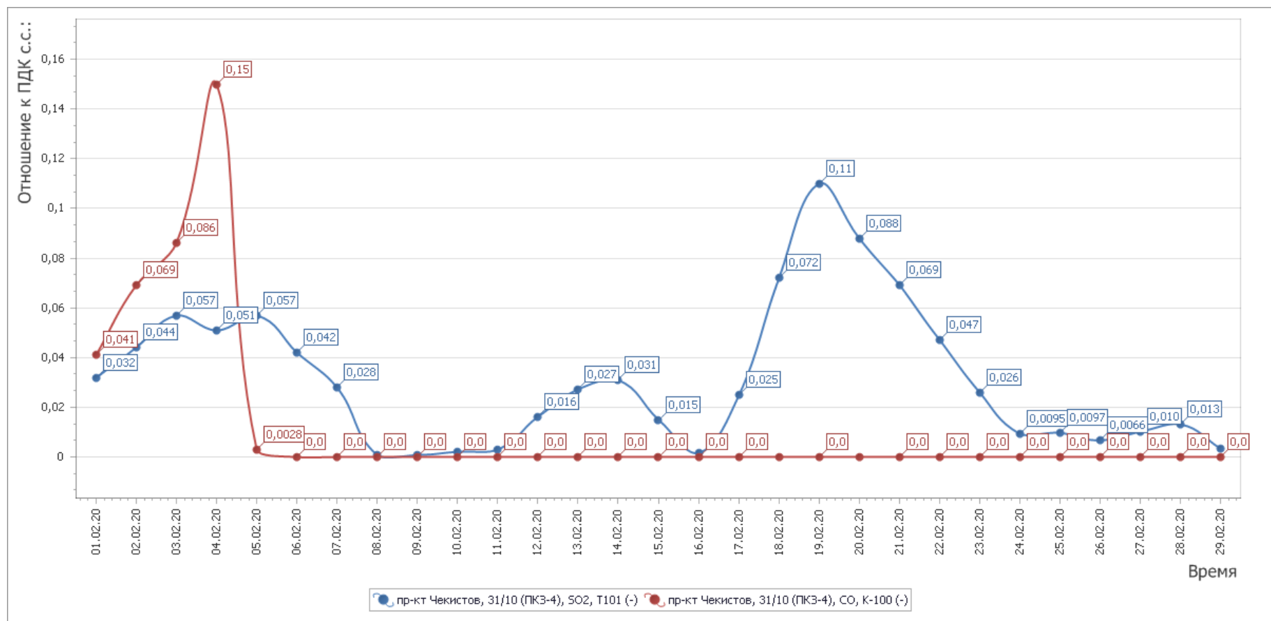
Рисунок 6 - График среднесуточных значений концентраций загрязняющих веществ (в долях ПДК) в атмосферном воздухе в период с 01.02.2020г. по 29.02.2020г. (ПКЗ 4 - автоматическая станция ул. Проспект Чекистов)
