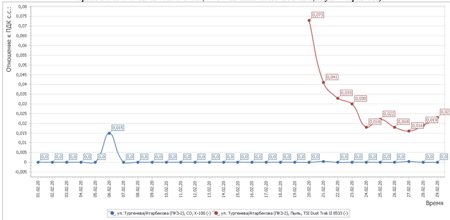
Рисунок 4 - График среднесуточных значений концентраций загрязняющих веществ (в долях ПДК) в атмосферном воздухе в период с 01.02.2020г. по 29.02.2020г. (ПКЗ-2 автоматическая станция ул. Атарбекова)
