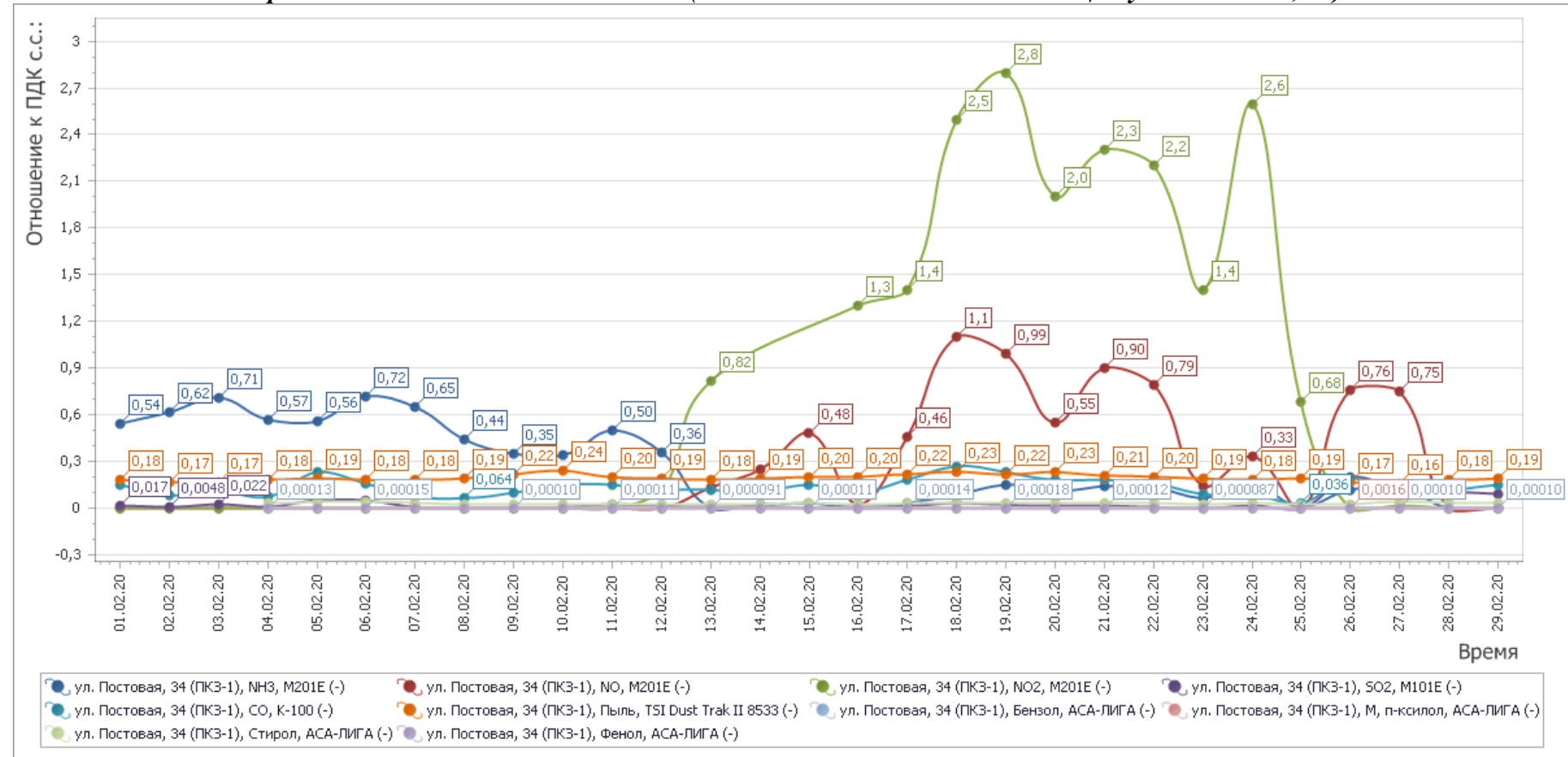
Рисунок 3- График среднесуточных значений концентраций загрязняющих веществ (в долях ПДК) в атмосферном воздухе в период с 01.02.2020г. по 29.02.2020г. (ПКЗ-1 - автоматическая станция ул. Постовая, 34)
