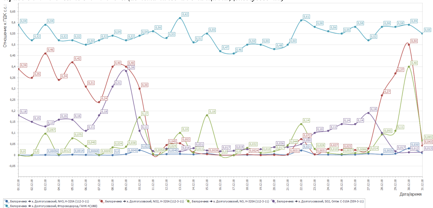
Рисунок 1- График среднесуточных значений концентраций загрязняющих веществ (в долях ПДК) в атмосферном воздухе в период с 01.12.2018г. по 31.12.2018 г. (автоматическая станция х. Долгогусевский)
