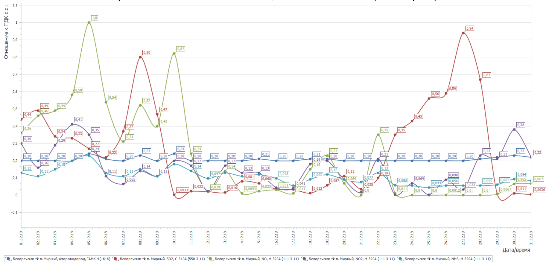
Рисунок 2- График среднесуточных значений концентраций загрязняющих веществ (в долях ПДК) в атмосферном воздухе в период с 01.12.2018г. по 31.12.2018 г. (автоматическая станция п. Мирный)
