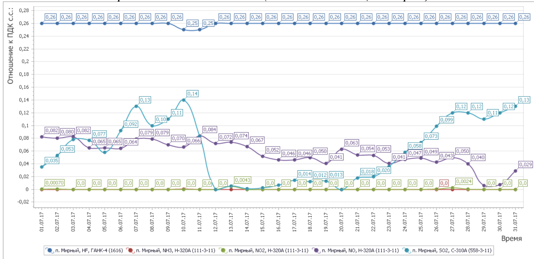
Рисунок 2- График среднесуточных значений концентраций загрязняющих веществ (в долях ПДК) в атмосферном воздухе в период с 01.07.2017г. по 31.07.2017 г. (автоматическая станция п. Мирный)
