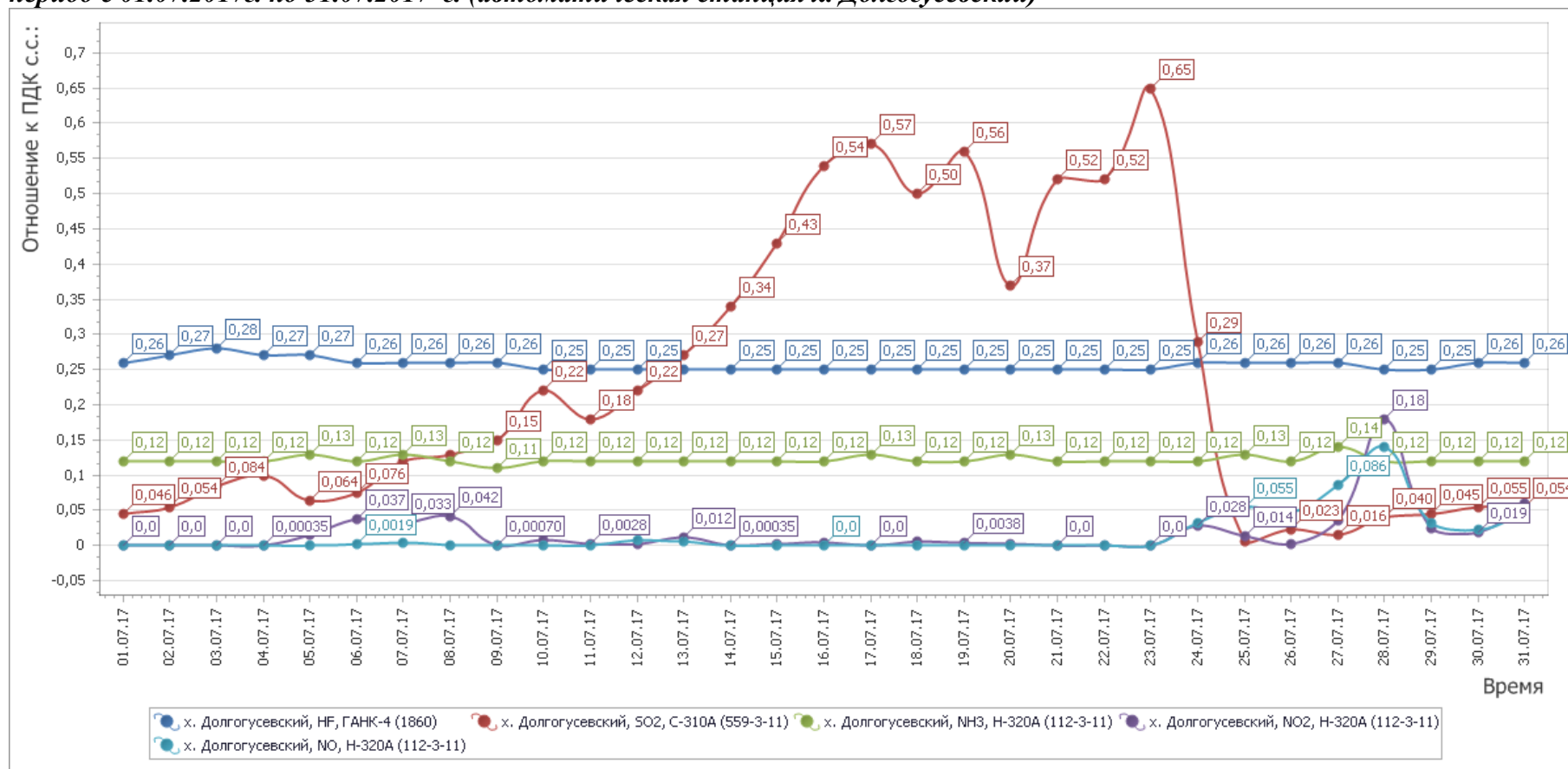
Рисунок 1- График среднесуточных значений концентраций загрязняющих веществ (в долях ПДК) в атмосферном воздухе в период с 01.07.2017г. по 31.07.2017 г. (автоматическая станция х. Долгогусевский)
