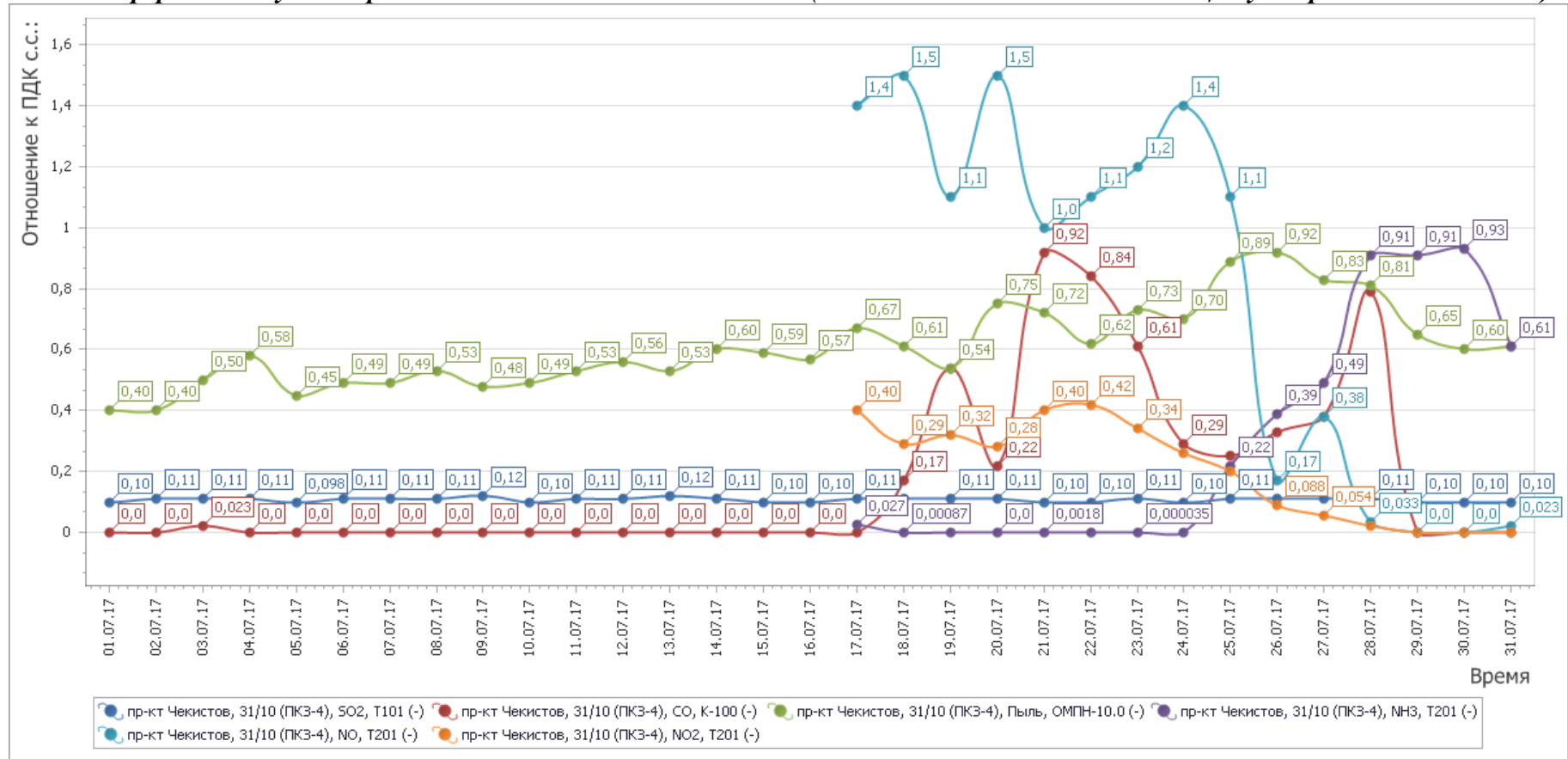
Рисунок 6 - График среднесуточных значений концентраций загрязняющих веществ (в долях ПДК) в атмосферном воздухе в период с 01.07.2017г. по 31.07.2017 г. (ПКЗ 4 - автоматическая станция ул. Проспект Чекистов)
