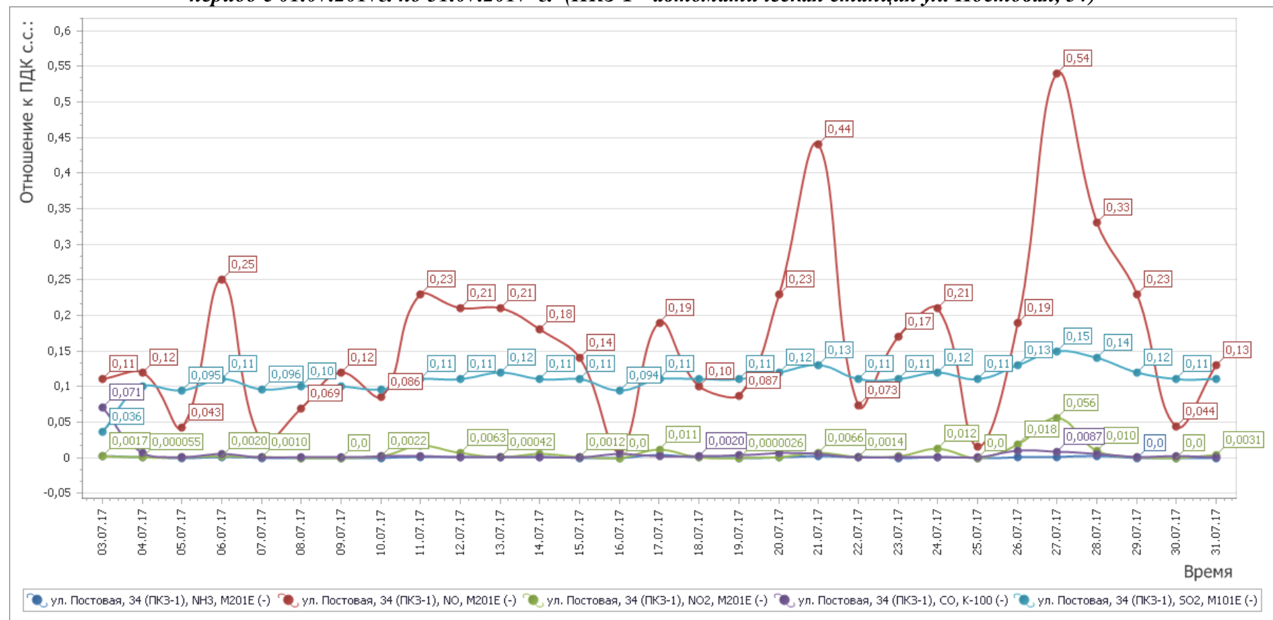
Рисунок 3- График среднесуточных значений концентраций загрязняющих веществ (в долях ПДК) в атмосферном воздухе в период с 01.07.2017г. по 31.07.2017 г. (ПКЗ-1 - автоматическая станция ул. Постовая, 34)
