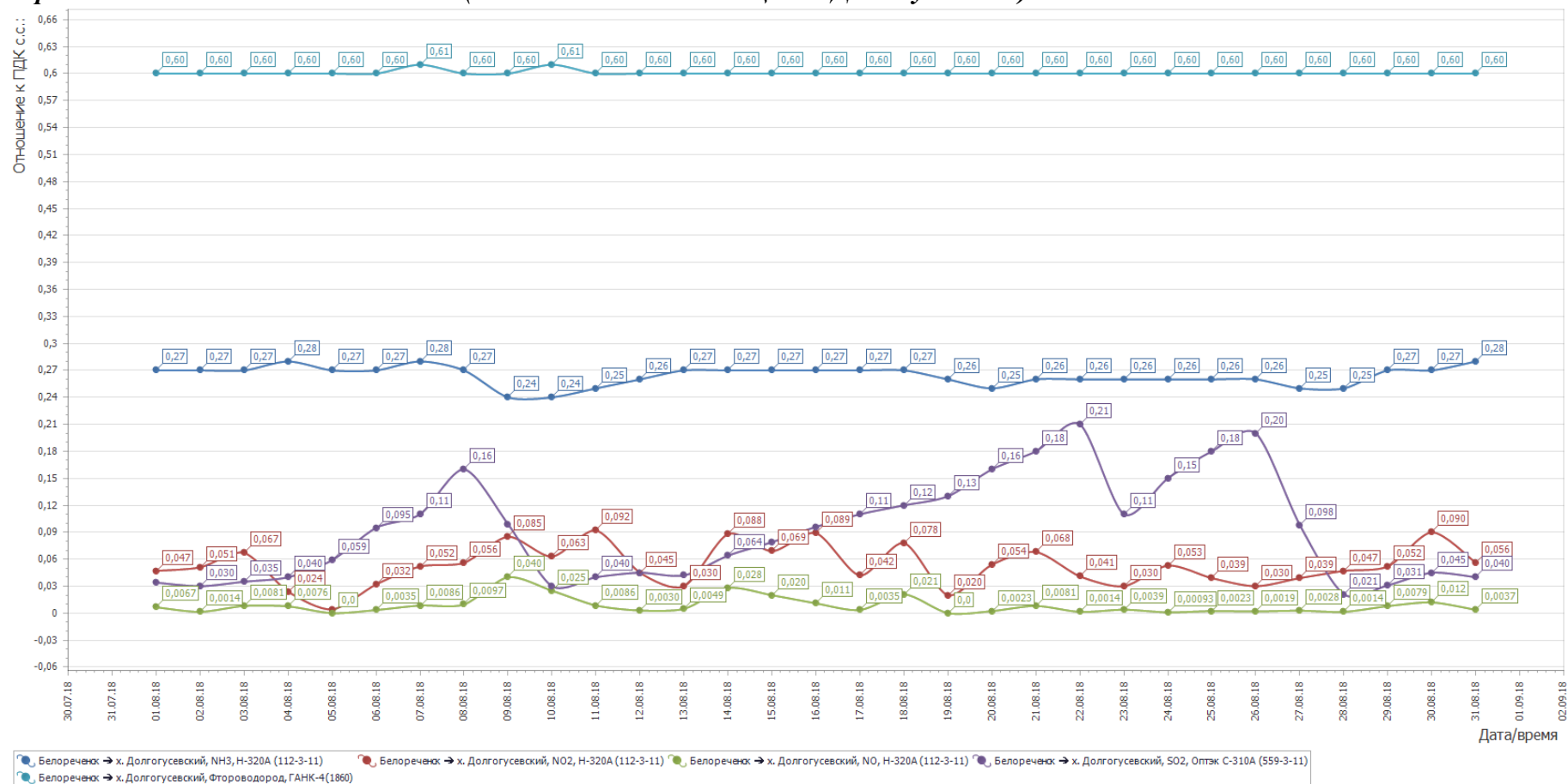
Рисунок 1- График среднесуточных значений концентраций загрязняющих веществ (в долях ПДК) в атмосферном воздухе в период с 01.08.2018г. по 31.08.2018 г. (автоматическая станция х. Долгогусевский)
