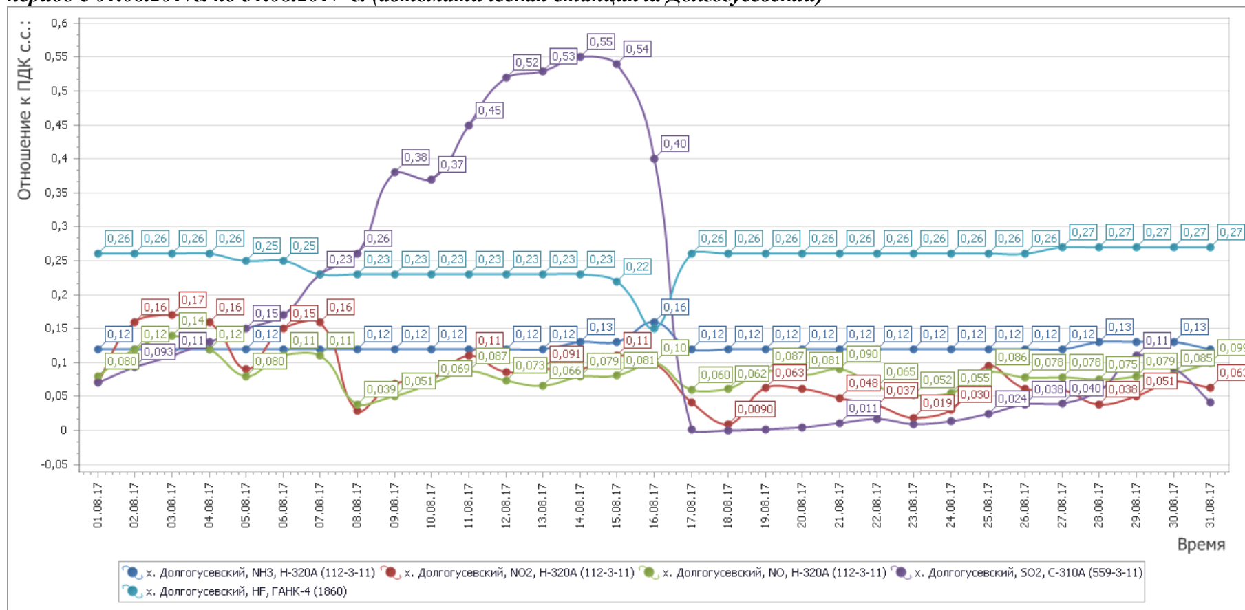
Рисунок 1- График среднесуточных значений концентраций загрязняющих веществ (в долях ПДК) в атмосферном воздухе в период с 01.08.2017г. по 31.08.2017 г. (автоматическая станция х. Долгогусевский)
