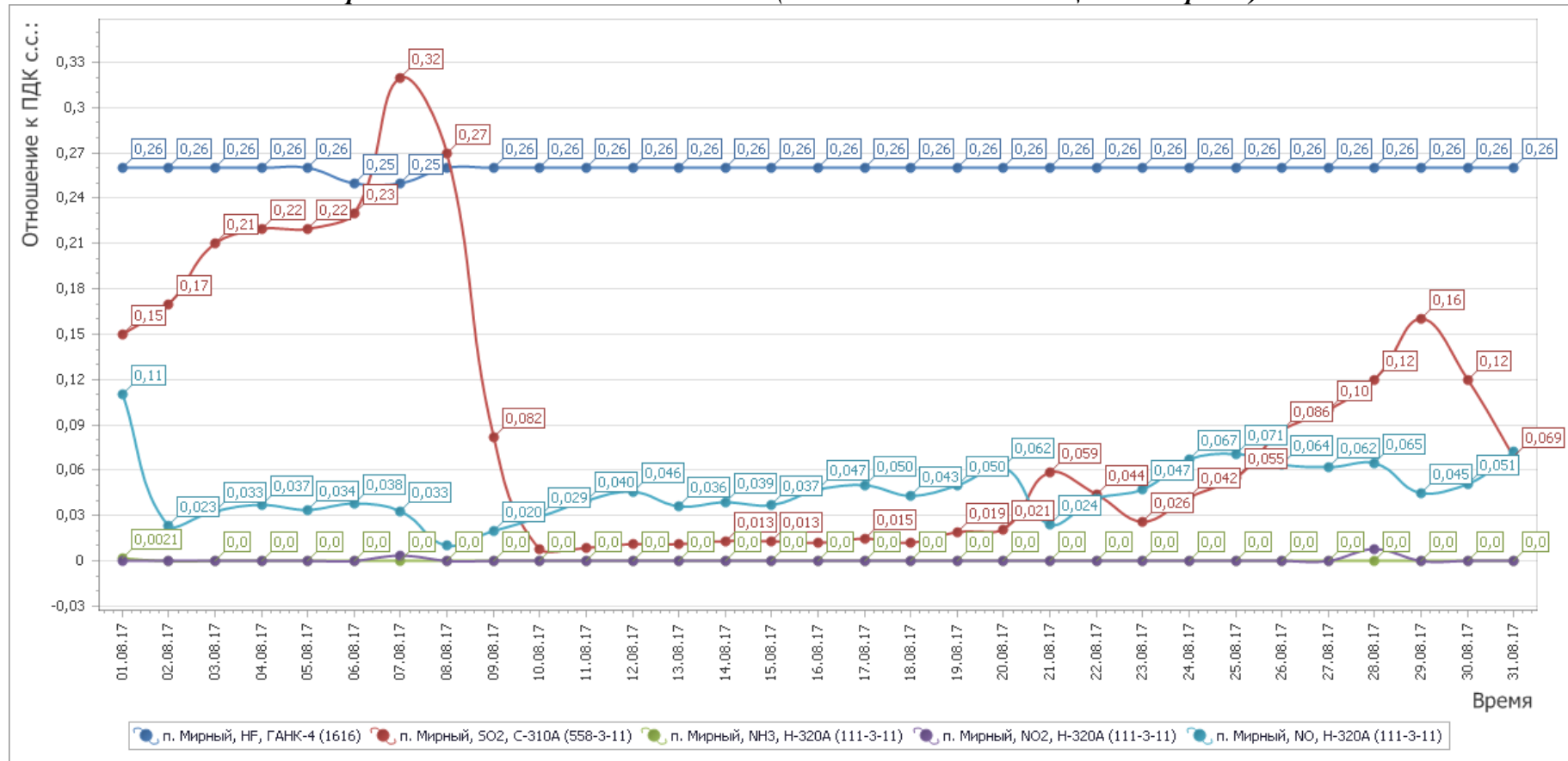
Рисунок 2- График среднесуточных значений концентраций загрязняющих веществ (в долях ПДК) в атмосферном воздухе в период с 01.08.2017г. по 31.08.2017 г. (автоматическая станция п. Мирный)
