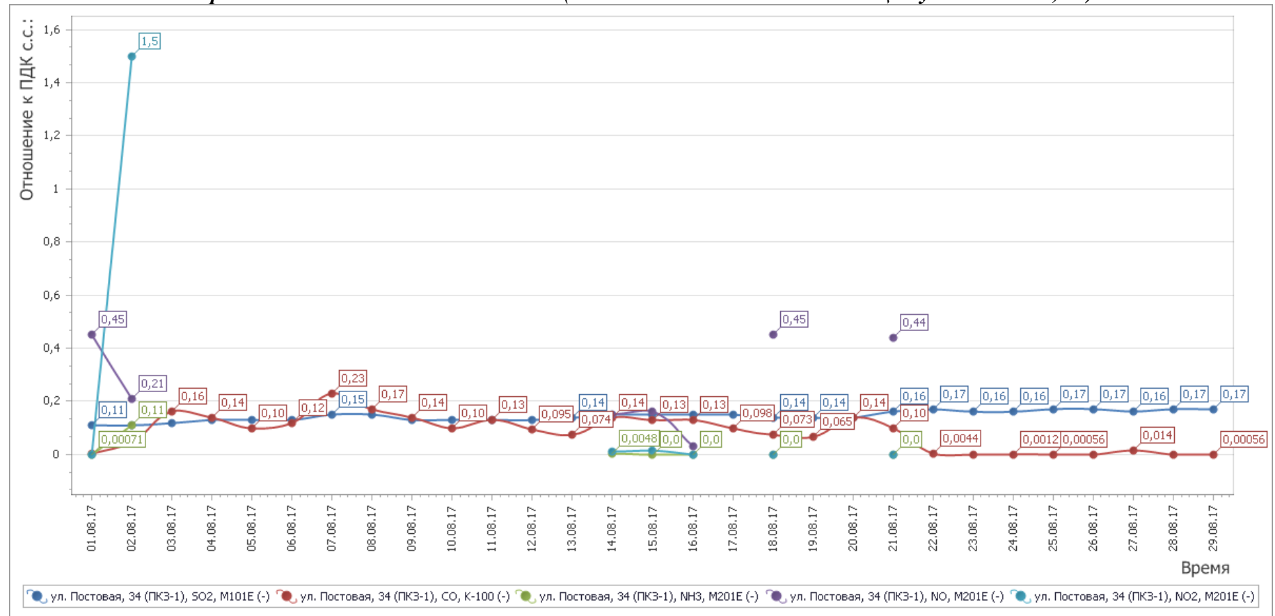
Рисунок 3- График среднесуточных значений концентраций загрязняющих веществ (в долях ПДК) в атмосферном воздухе в период с 01.08.2017г. по 31.08.2017 г. (ПКЗ-1 - автоматическая станция ул. Постовая, 34)
