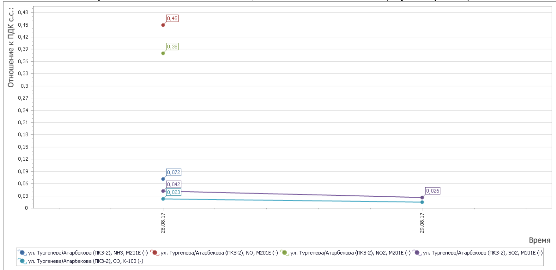
Рисунок 4 - График среднесуточных значений концентраций загрязняющих веществ (в долях ПДК) в атмосферном воздухе в период с 01.08.2017г. по 31.08.2017 г. (ПКЗ-2 автоматическая станция ул. Атарбекова)
