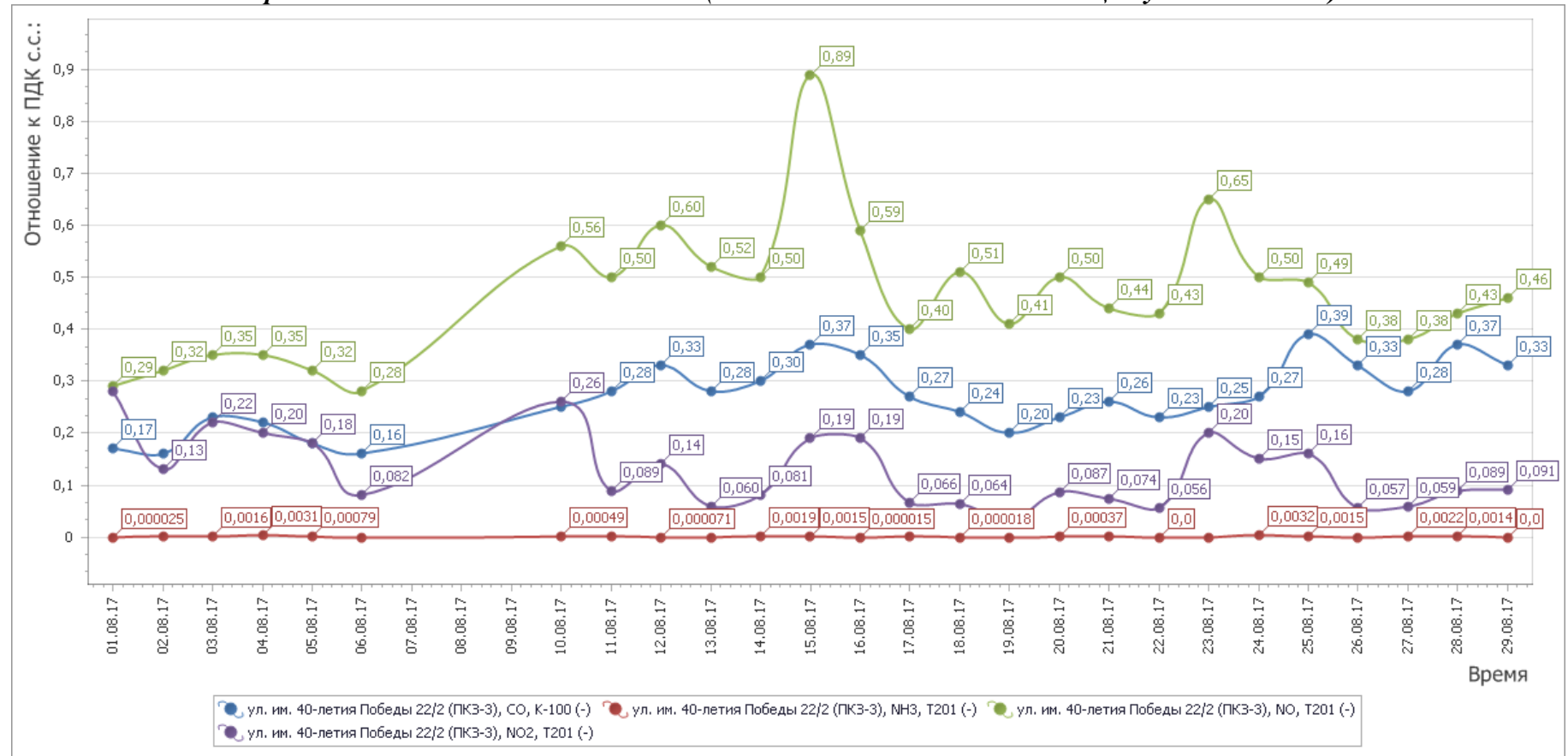
Рисунок 5 - График среднесуточных значений концентраций загрязняющих веществ (в долях ПДК) в атмосферном воздухе в период с 01.08.2017г. по 31.08.2017 г. (ПКЗ-3 - автоматическая станция ул. Московская)
